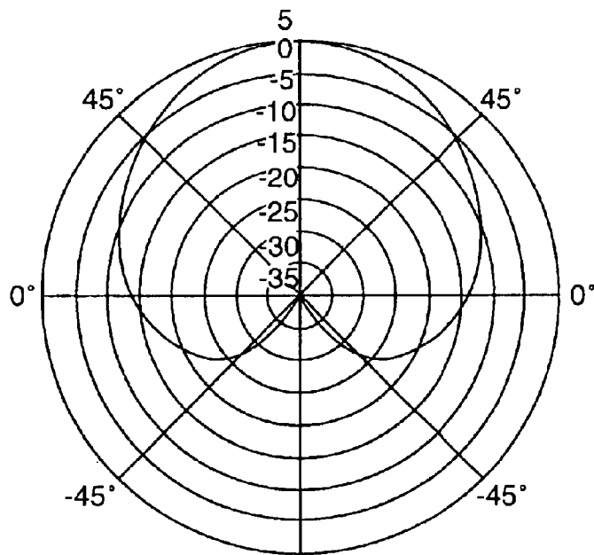
FIG. 6 GAIN (dBiRC)
