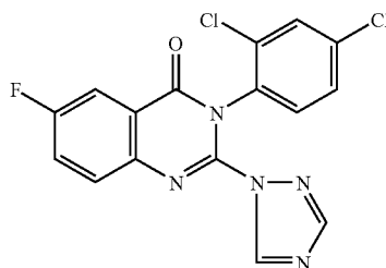
(FLUQUINCONAZOLE)
