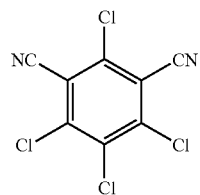
(CHLOROTHALONIL)
