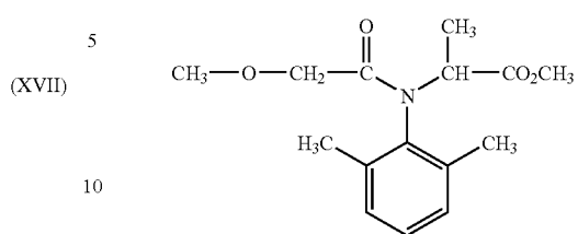
(METALAXYL)
