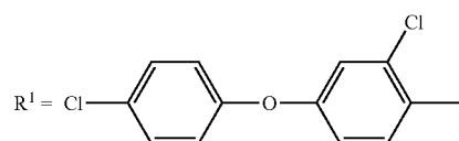
(DIFENCONAZOLE)
