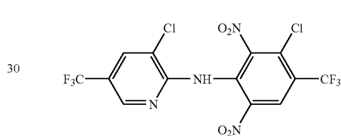
(FLUAZINAM)
