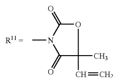
(VINCLOZOLIN) (XIV-1)
