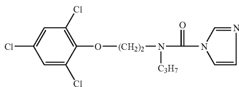
(PROCHLORAZ)
