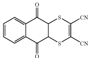
(DITHIANON)
