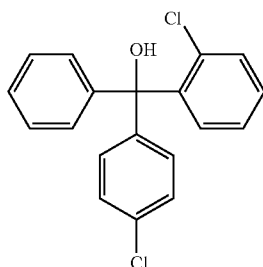
(FENARIMOL)
