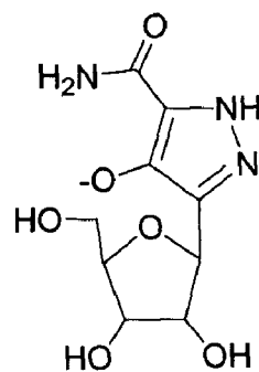
Pyrazofurin (14)
