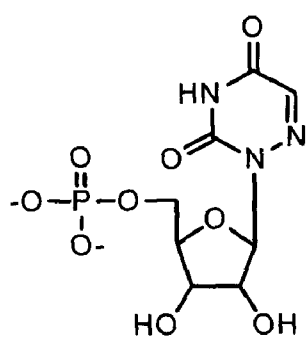
6-Aza-UMP
