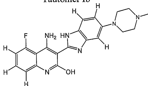
Tautomer Ic
