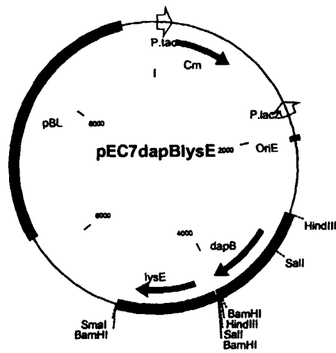
Abbildung 3: Plasmid pEC7dapBlysE
