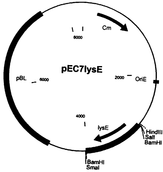
Abbildung 1: Plasmid pEC7lysE
