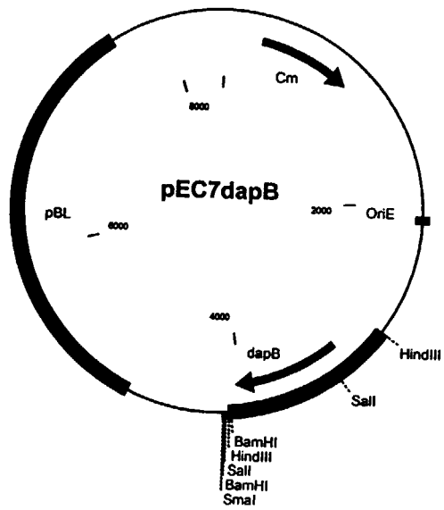
Abbildung 2: Plasmid pEC7dapB
