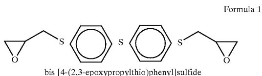
bis [4-(2,3-epoxypropylthio)phenyl]sulfide
