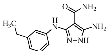
5-amino-3-((3-ethylphenyl)amino)-1 H -pyrazole-4-carboxamide
