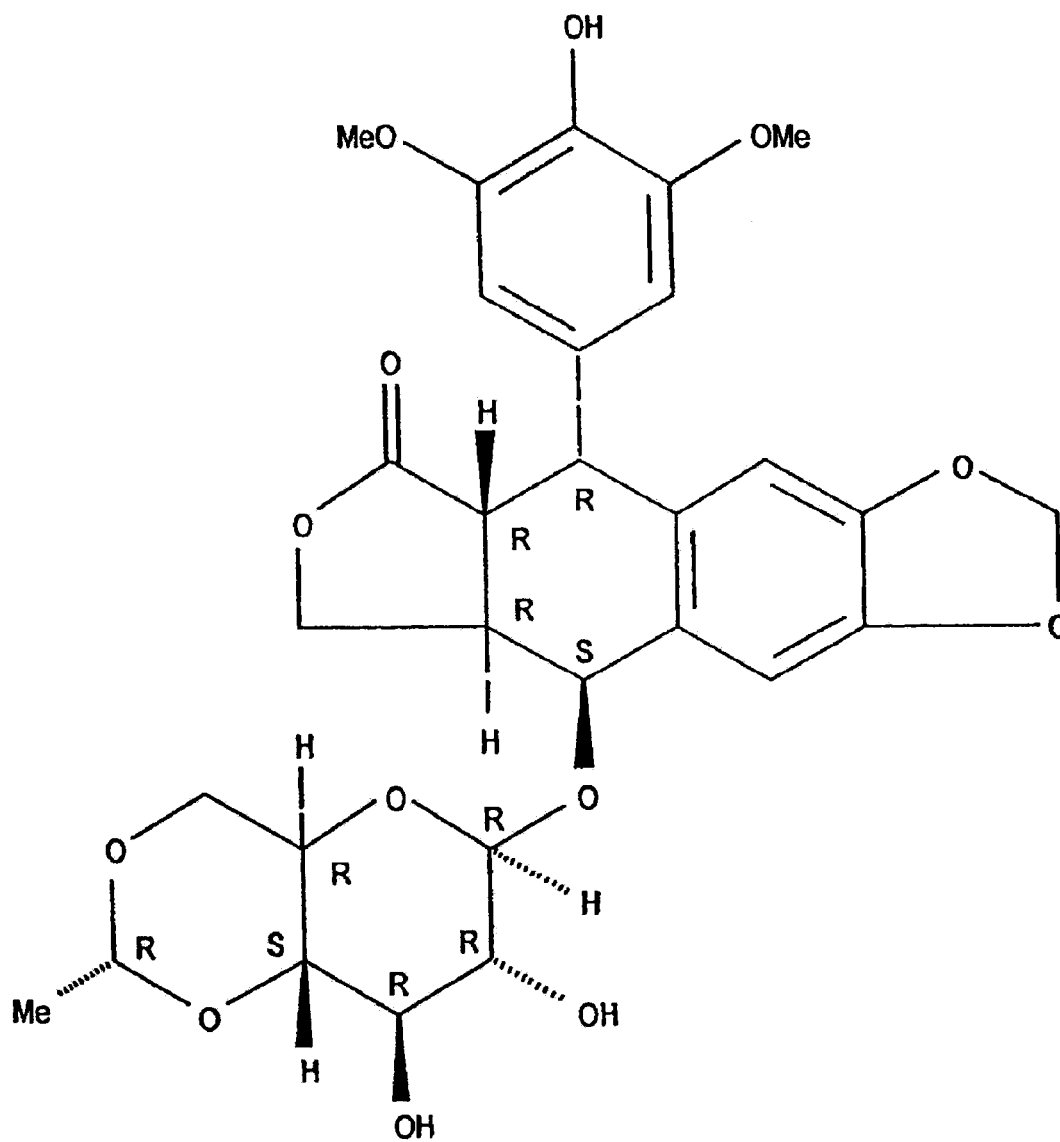
Etoposide (2)
