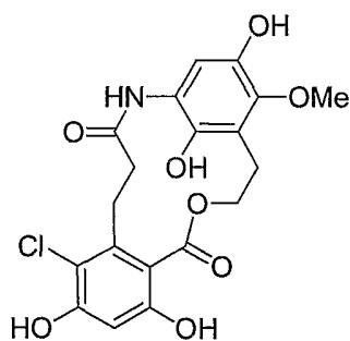
1,4 DIOL
