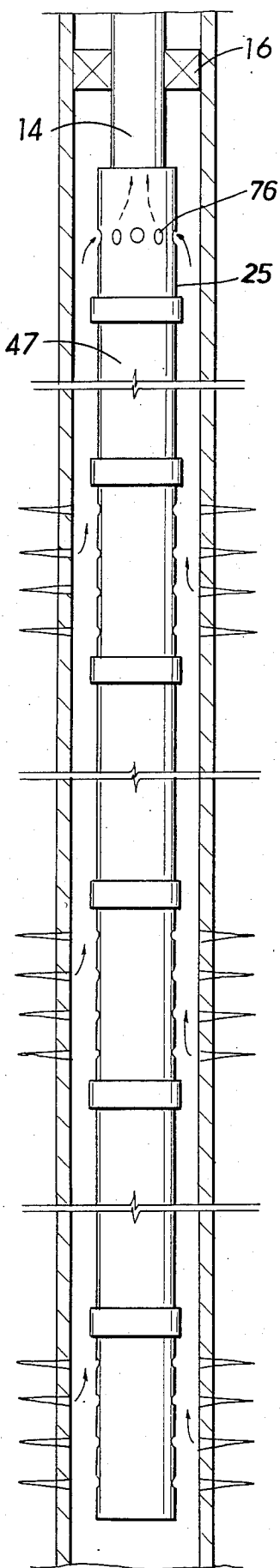
FIG. 7
