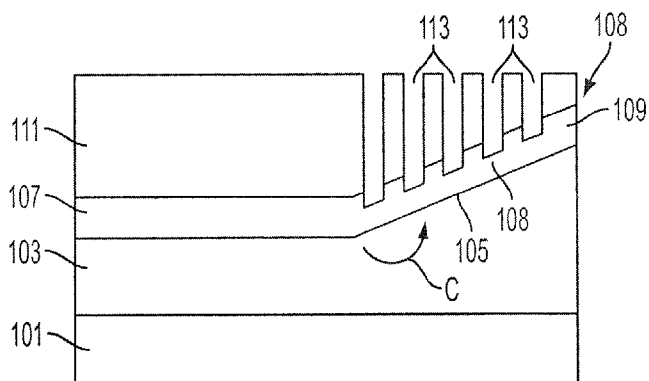
FIG. 3H
