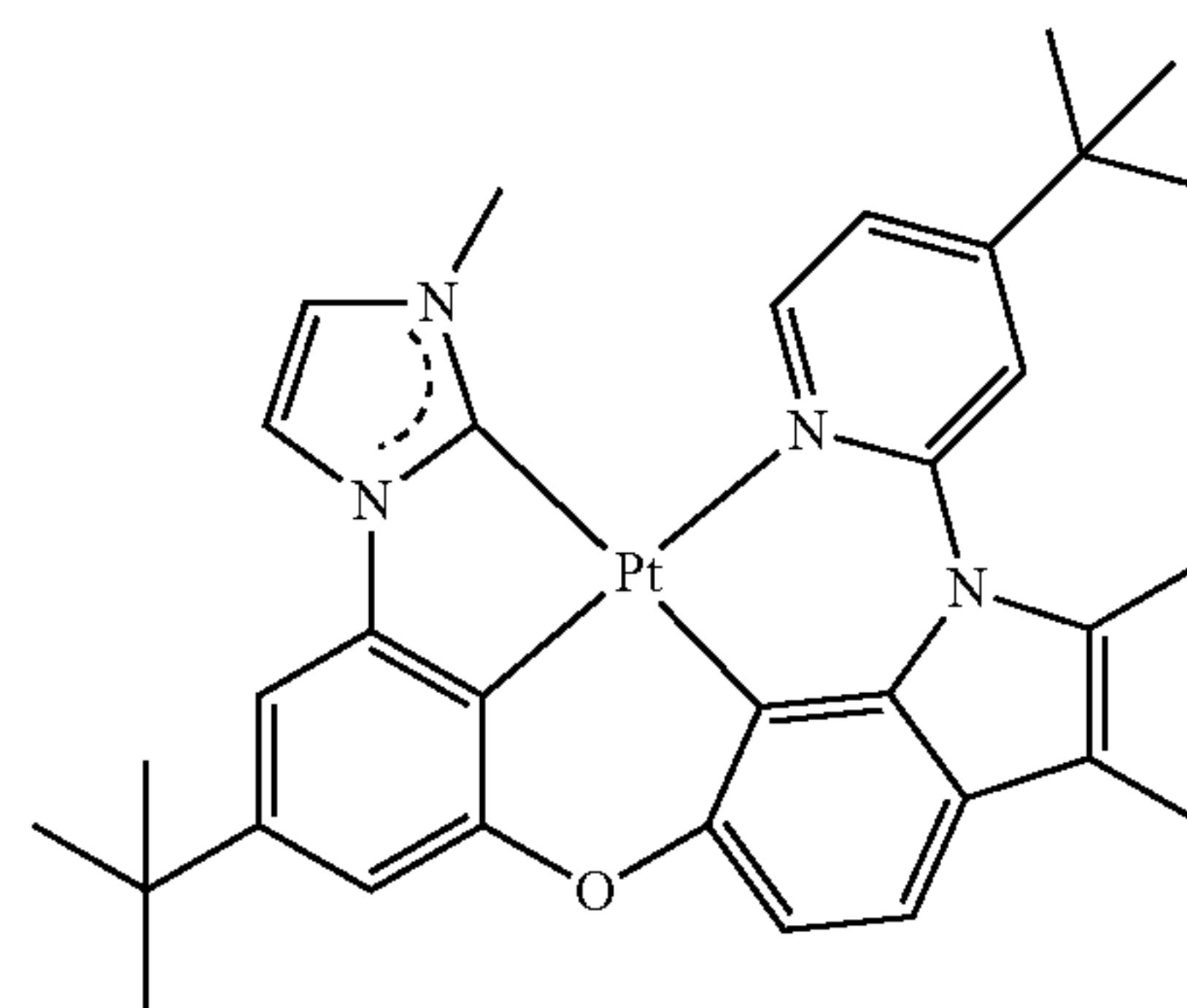
PtON7-dtb
