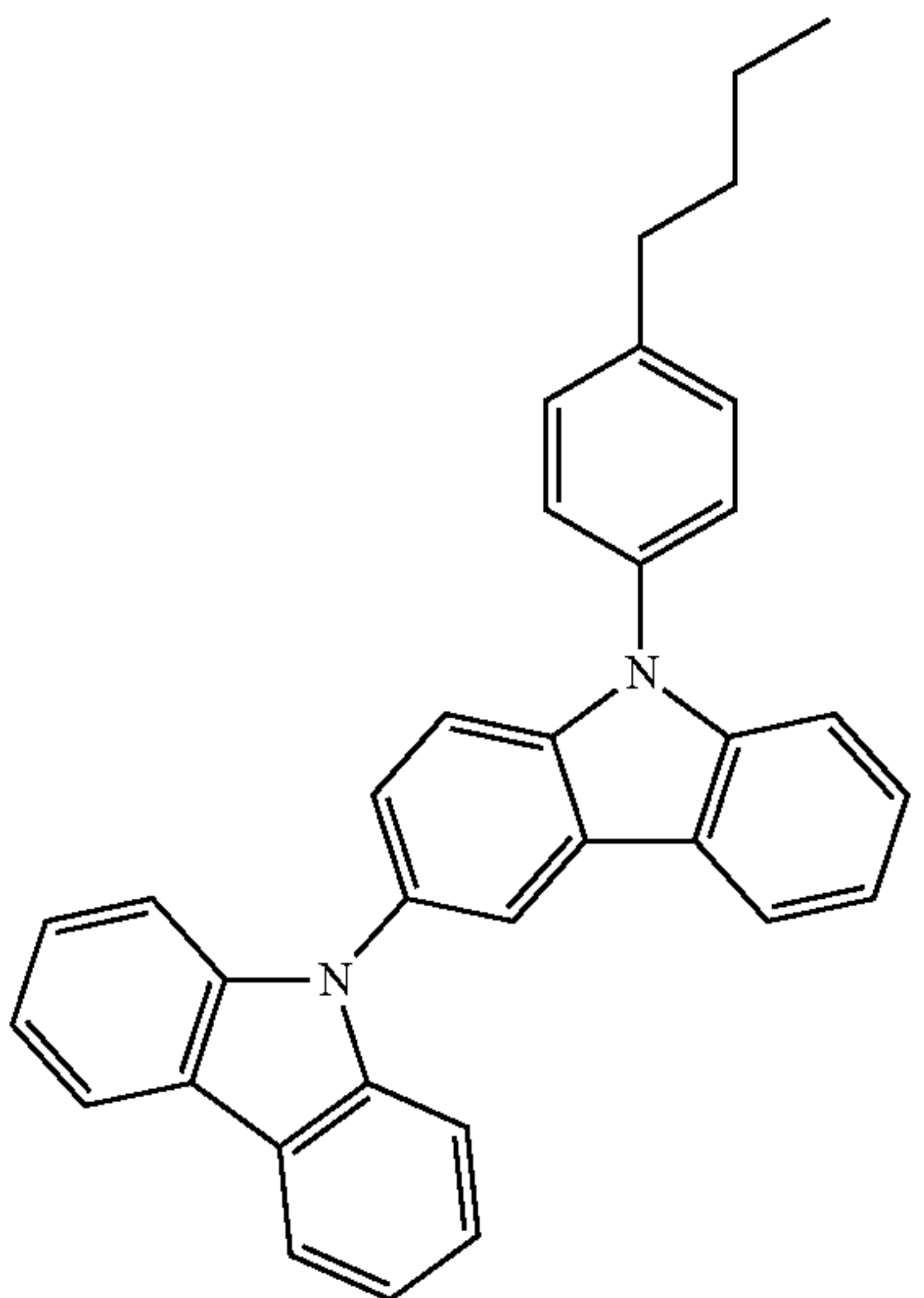
BCz2
