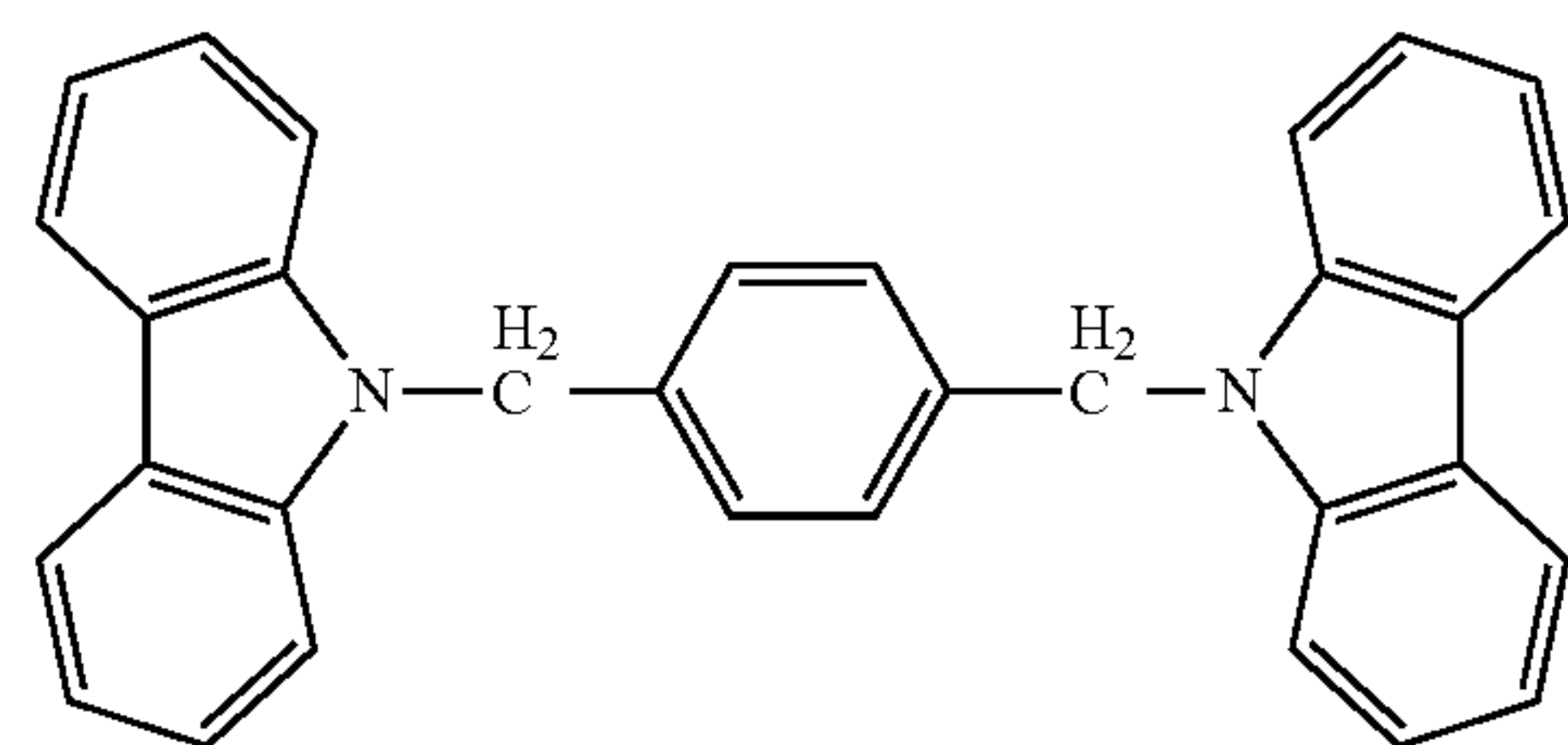
TCz2
