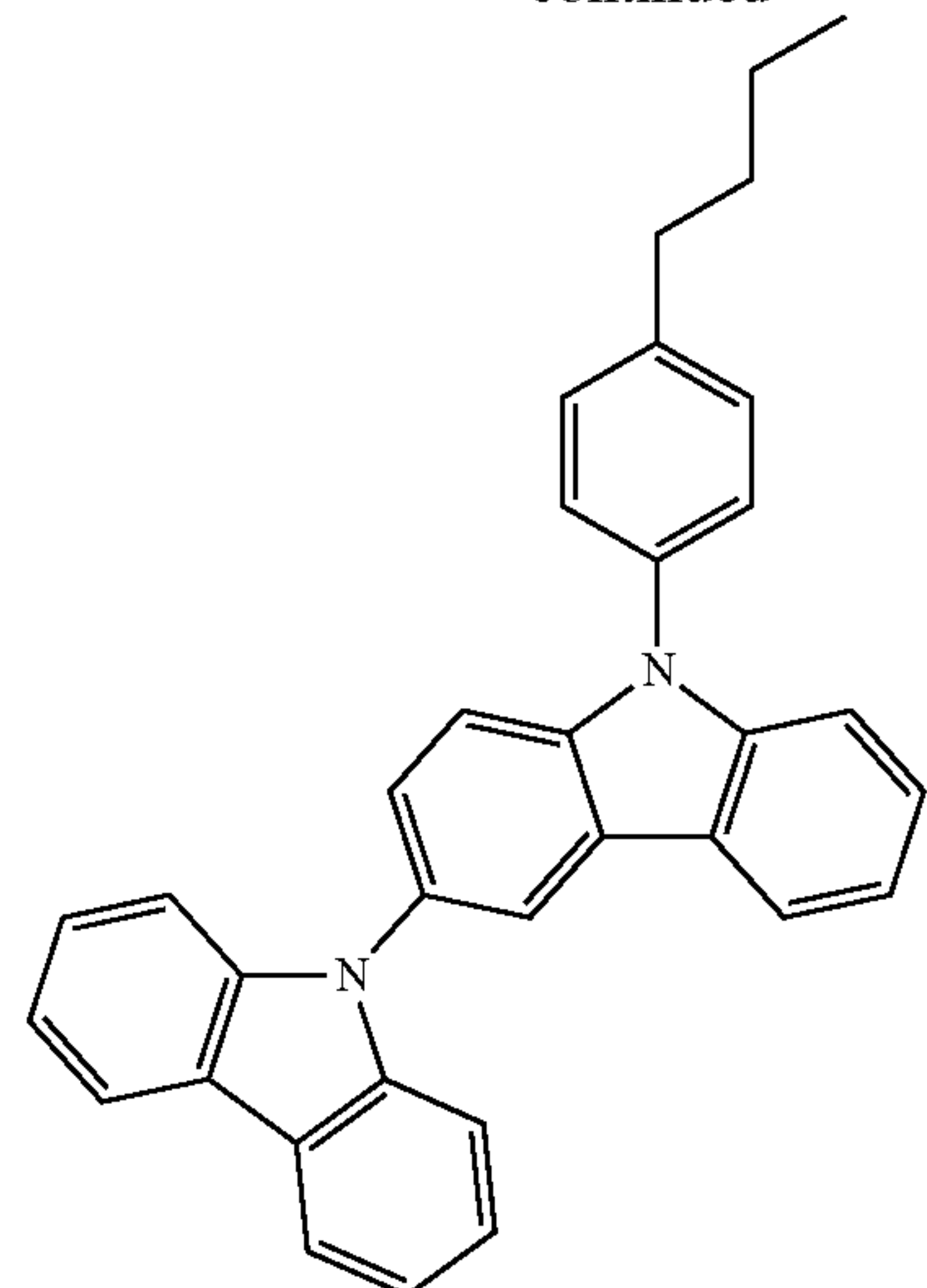
BCz2
