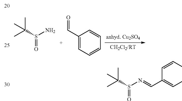
(R,E)-N-benzylidene-2-methylpropane-2-sulfinamide
