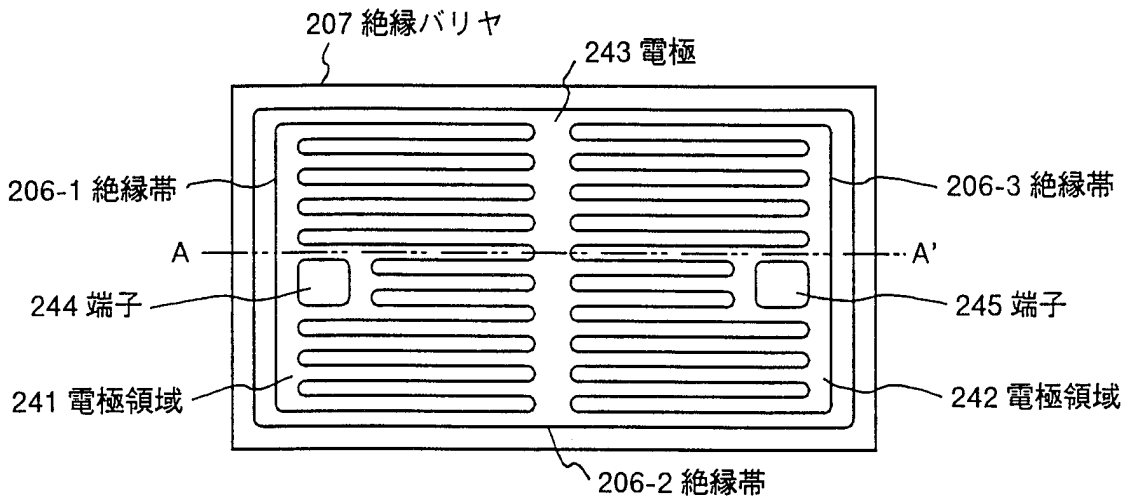
(a) 平面図
