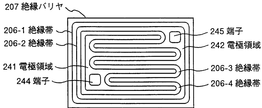
(b) 2重絶縁
