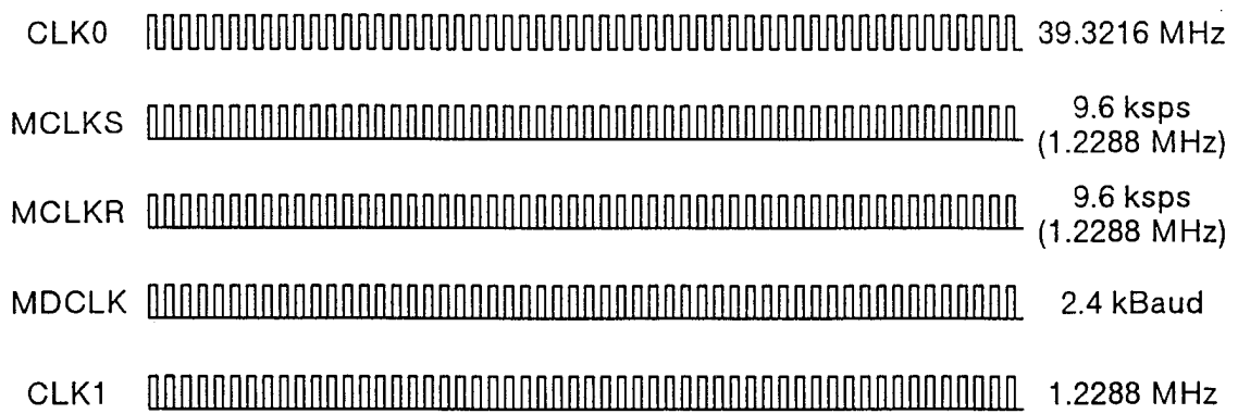
(a) モデム信号処理部分
