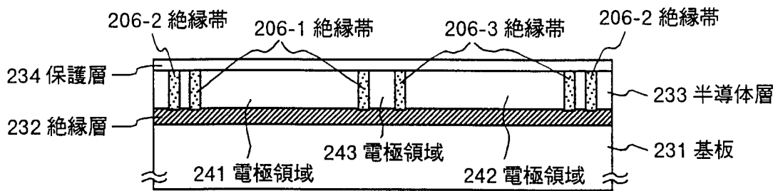
(b) 内層1層タイプの(A-A')断面図
