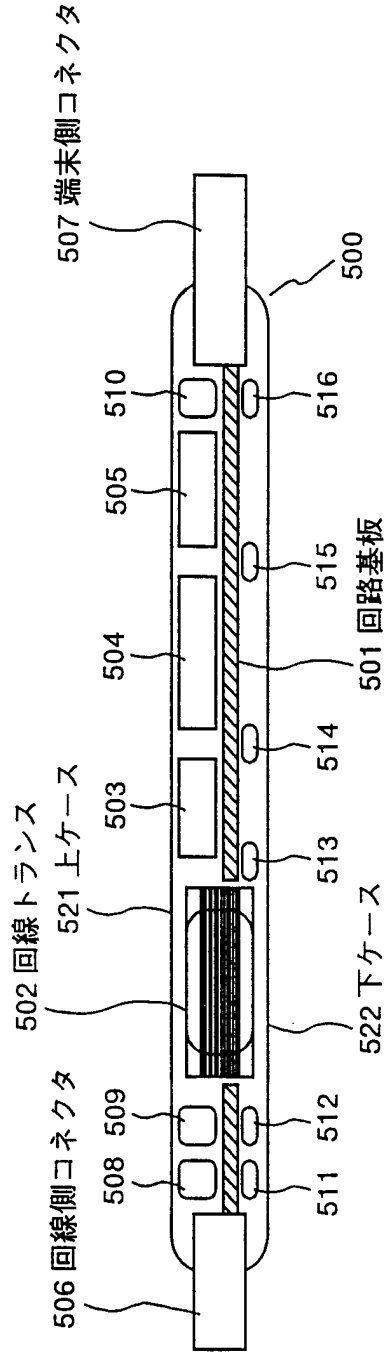
(b) 従来のモデム装置の構造
