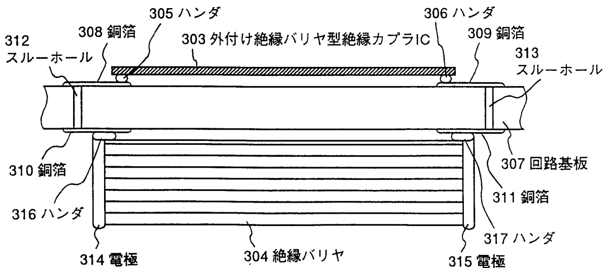
(b) 回路基板実装断面図
