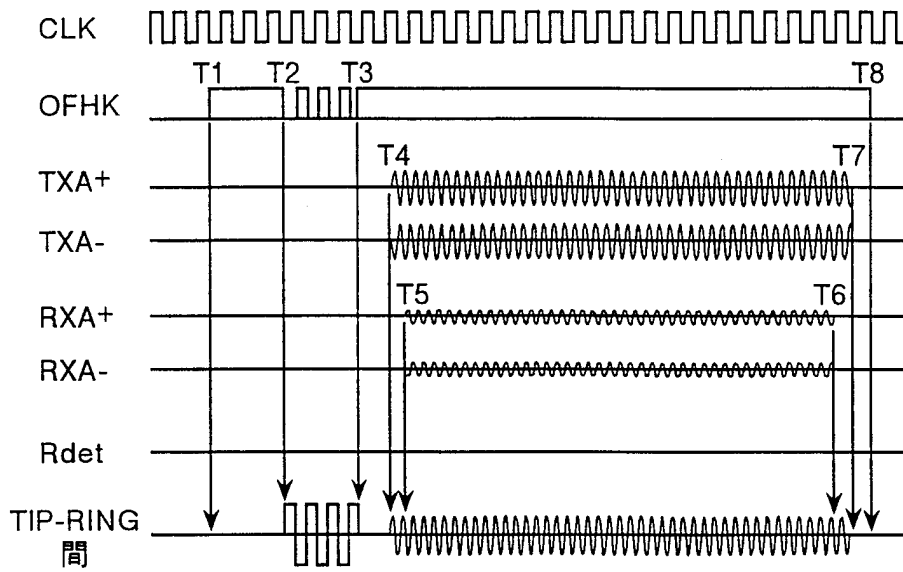
(a) 送信時の動作
