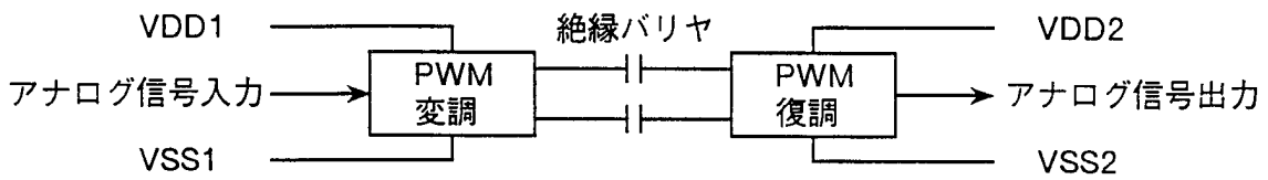
(b) PWM伝送方式
