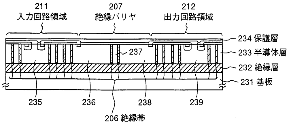
(b) 絶縁カプラの断面図
