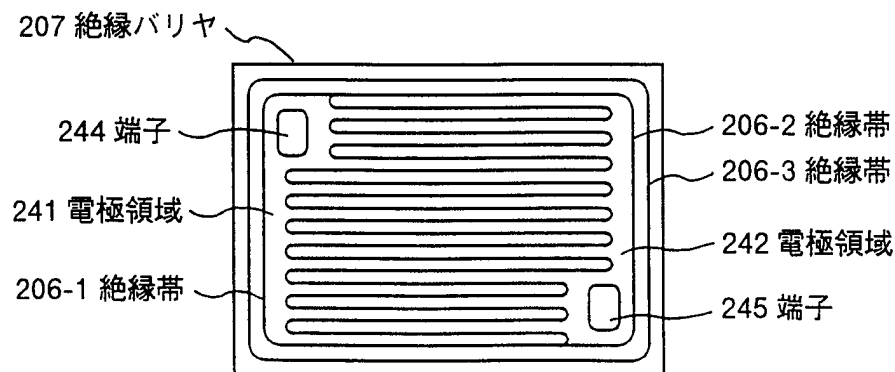
(c) (a) の変形例
