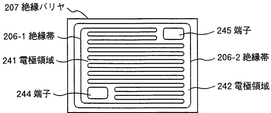
(a) 1重絶縁
