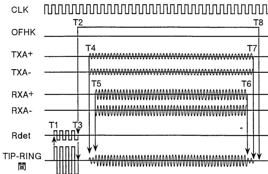
(b) 受信時の動作
