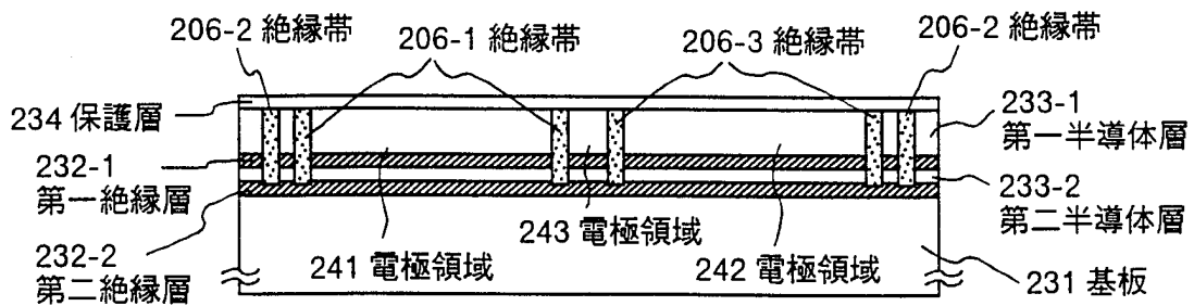
(c) 内層2層タイプの(A-A')断面図
