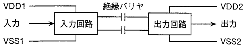
(b) PWM伝送方式
