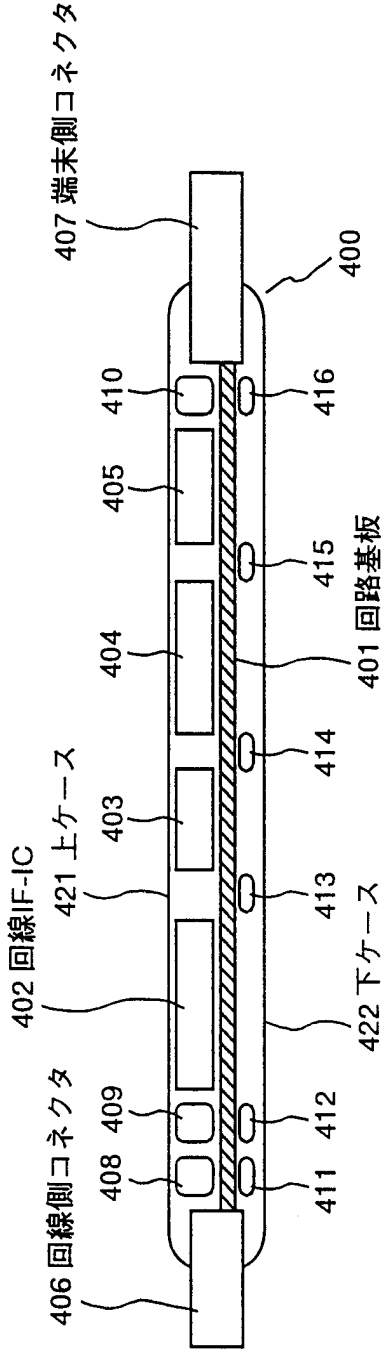
(a) 本発明の実施例の構造
