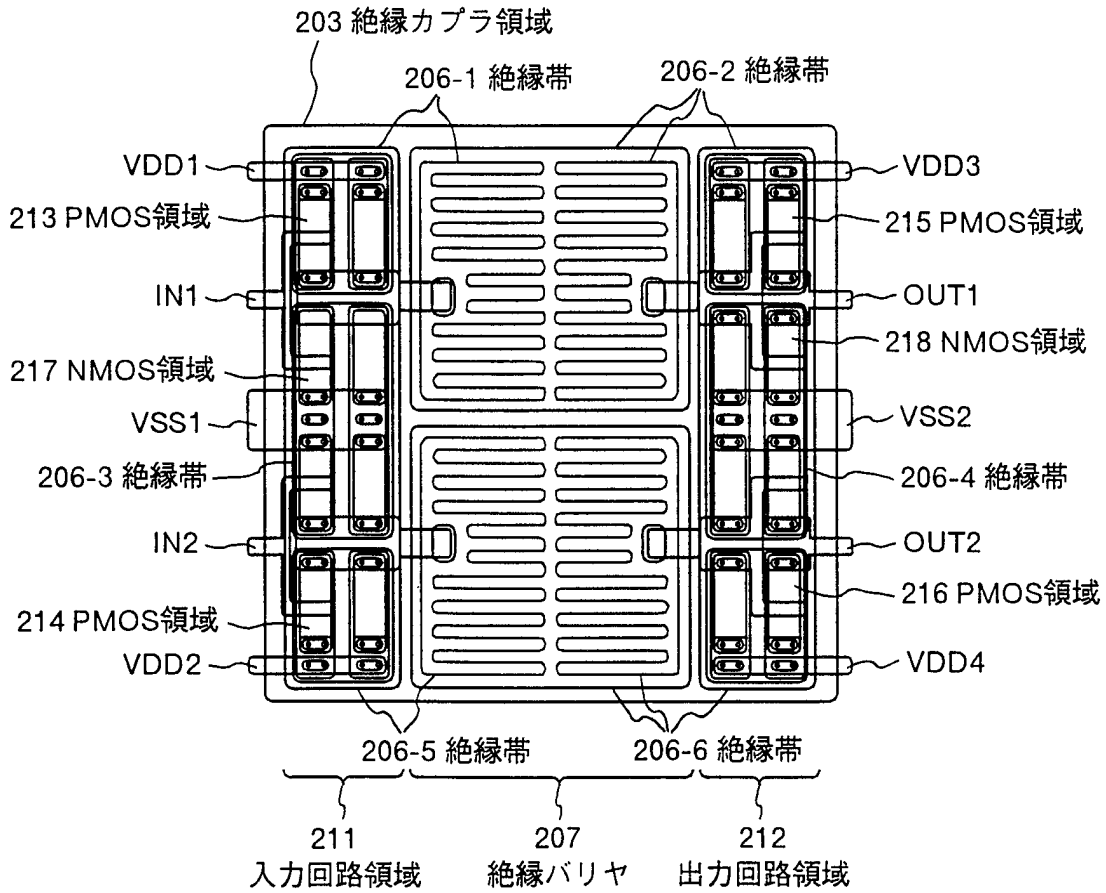
(a) 絶縁カプラの平面図
