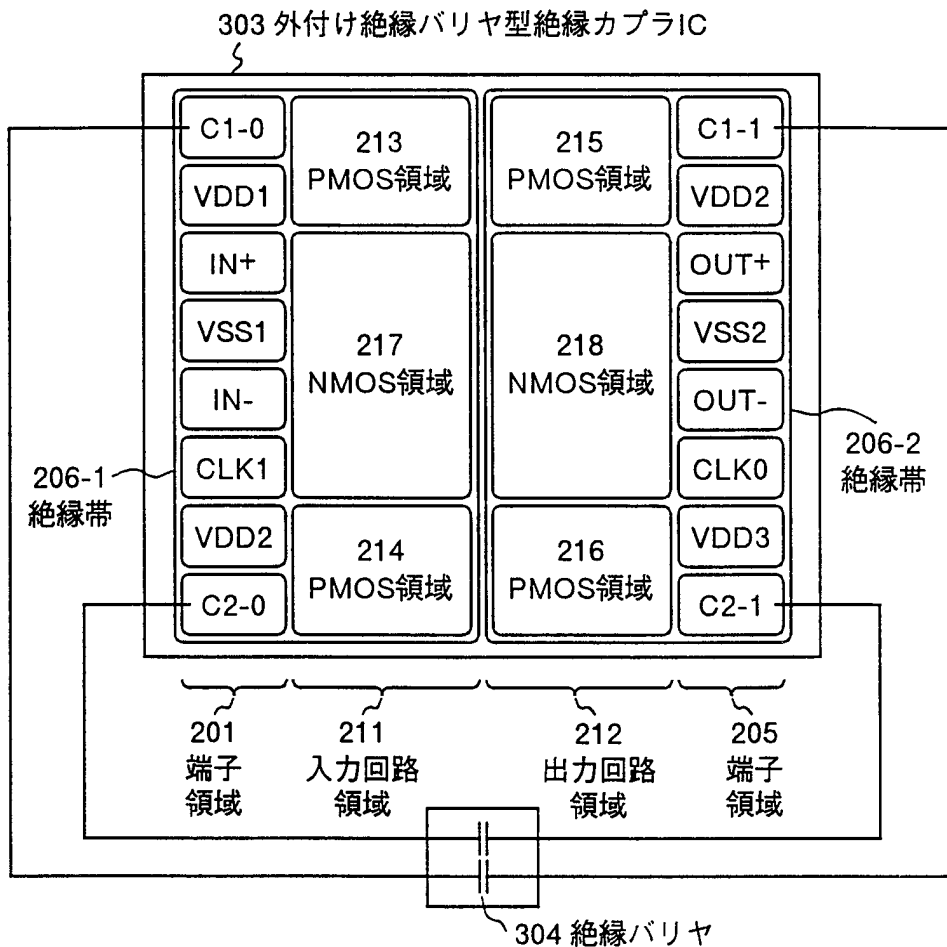
(a) チップレイアウト概要
