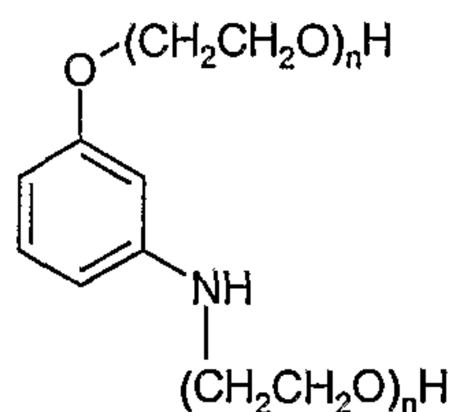
di-PEG 3-aminophenol
