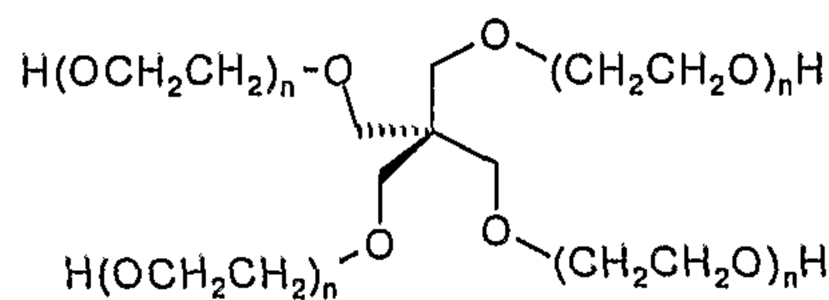
tetra-PEG-pentaerythritol
