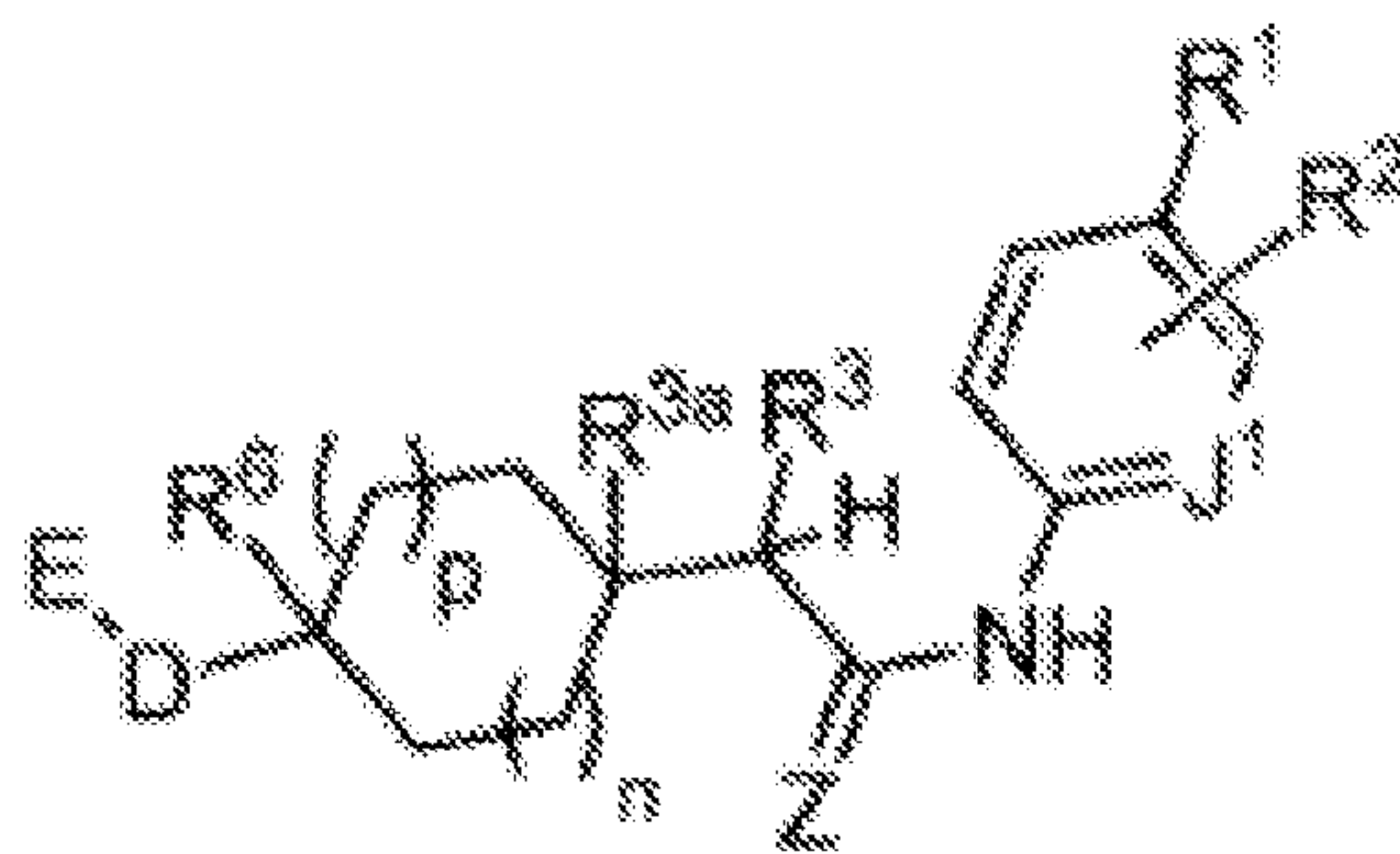
Formula (LIVh);
