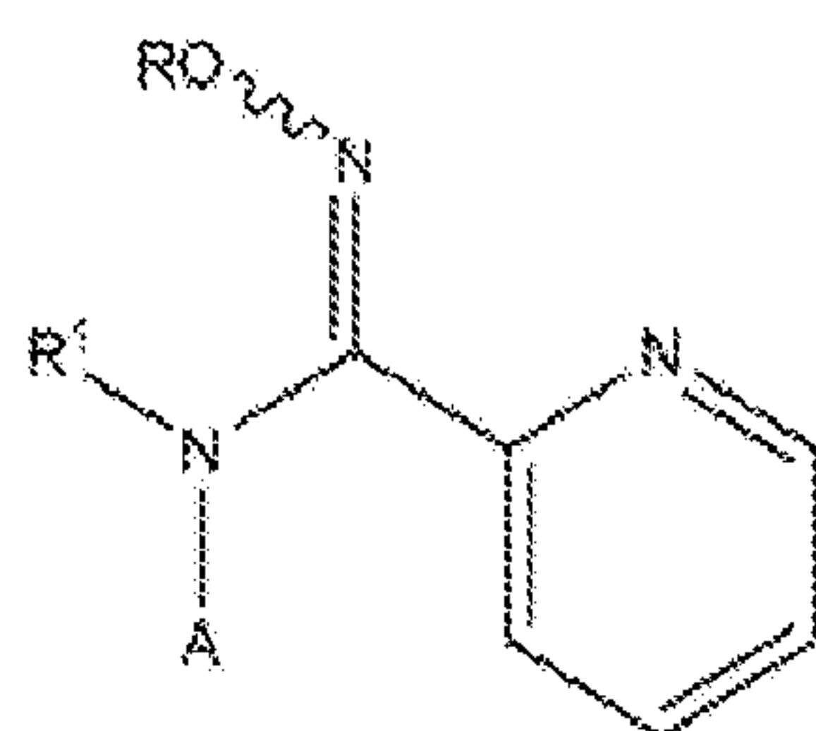
Formula (XVIIe);
