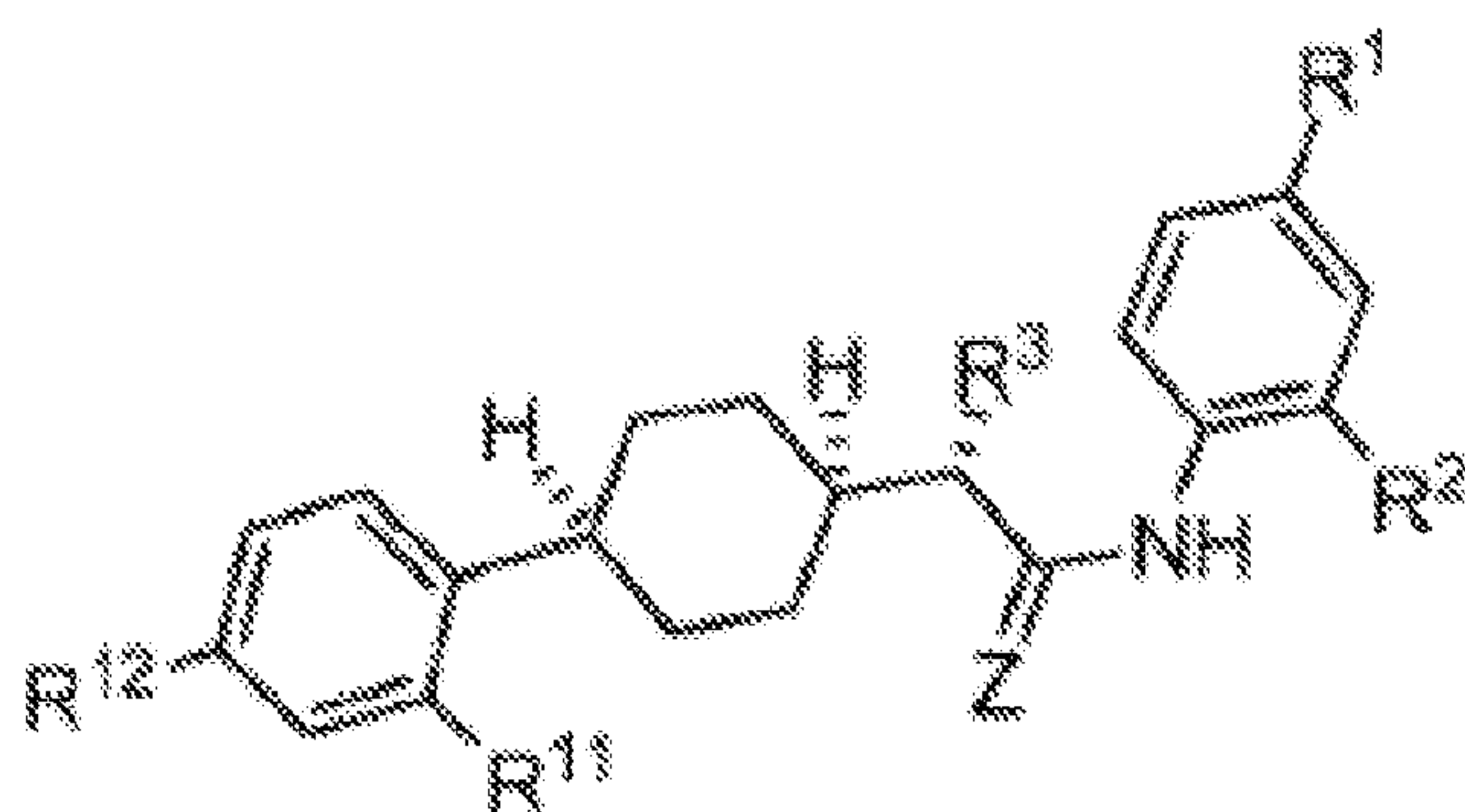
Formula (LIVaa).
