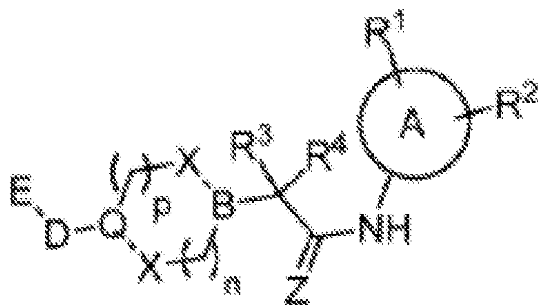
Formula (LIV).
