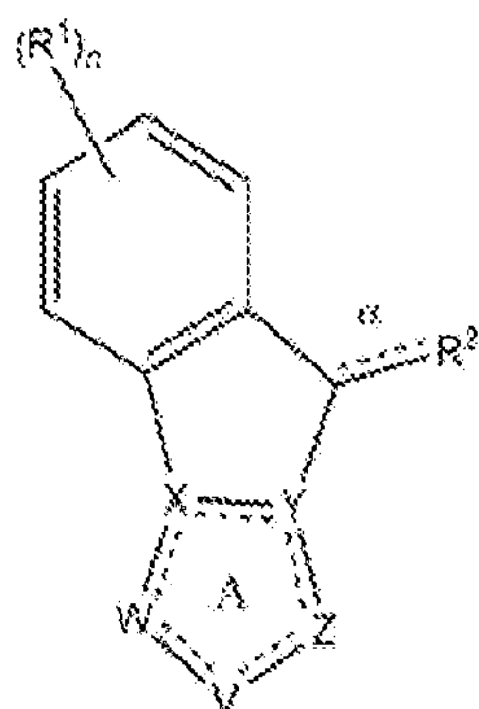
Formula (XXIX).
