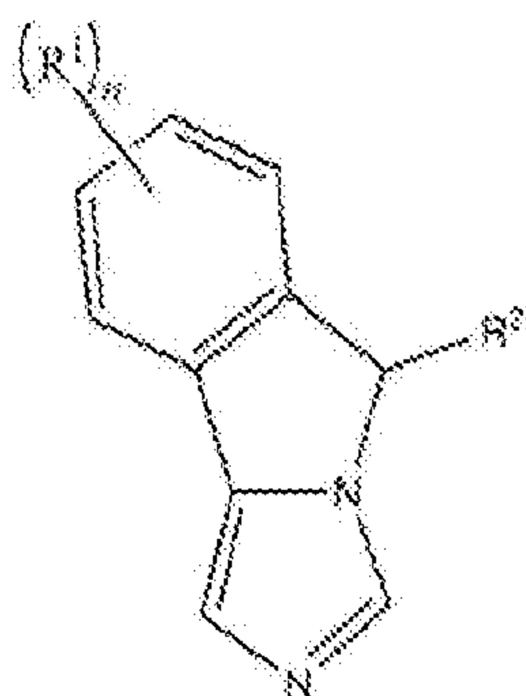
Formula (Xa);
