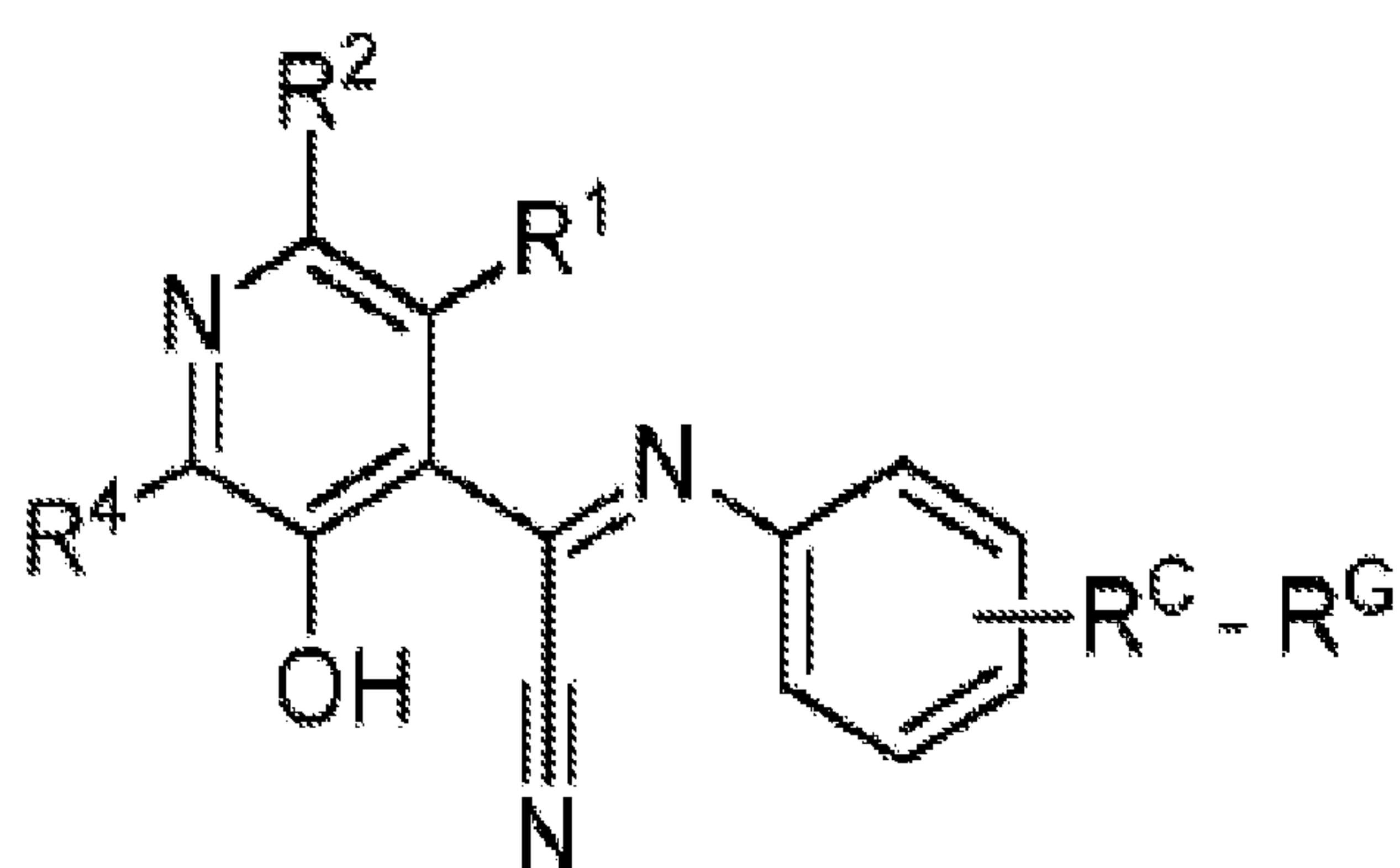
Formula (XLVIa);
