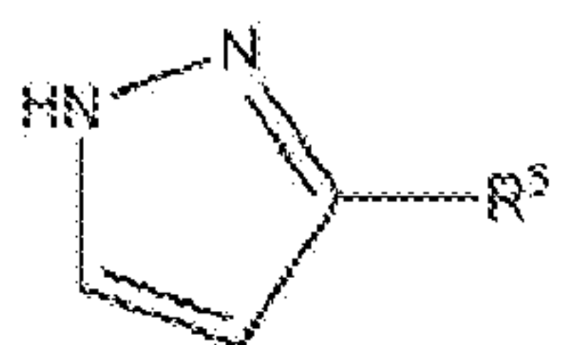
Formula (IXao);
