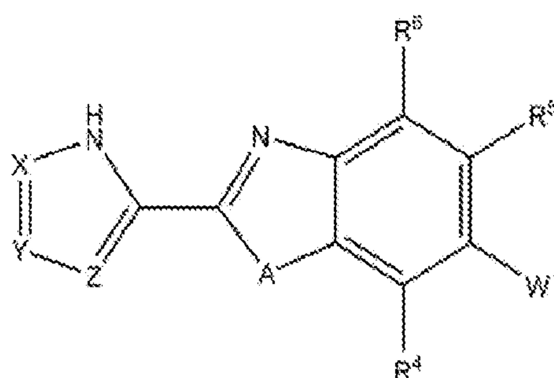
Formula (XIX).
