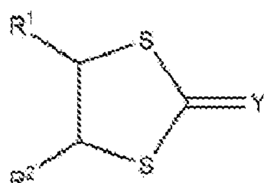
Formula (XXVIId);
