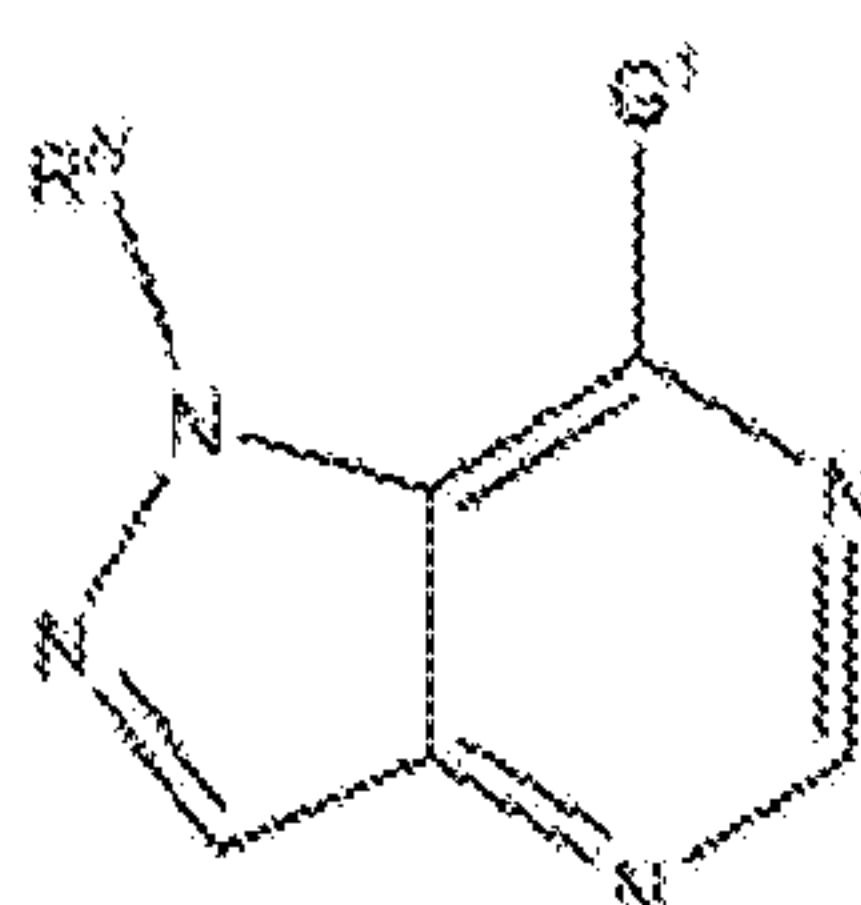
Formula (XXVIIIk);
