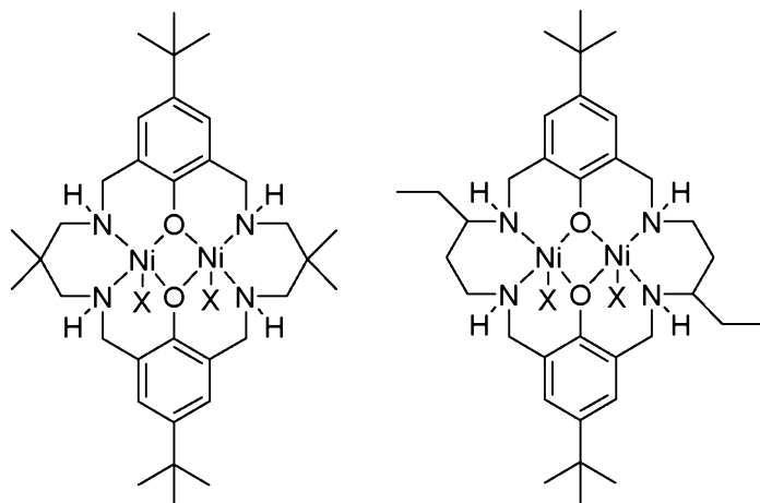
L^1Ni_2X_2 X = O_2CCF_3 X = O_2C(CH_2)_3Cy
