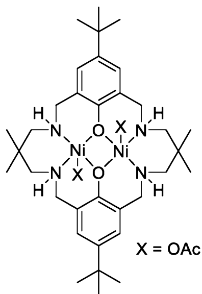
[L^1Ni_2(OAc)_2]
