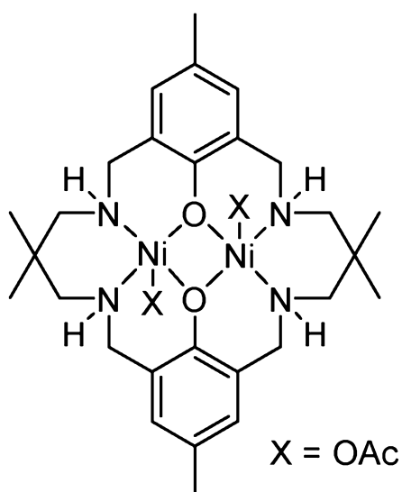
[L^2Ni_2(OAc)_2]
