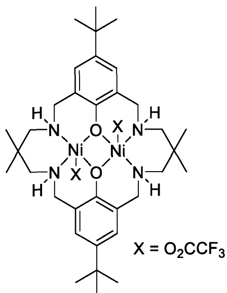
[L^1Ni_2(O_2CCF_3)_2]
