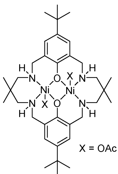
[L^1Ni_2(OAc)_2]
