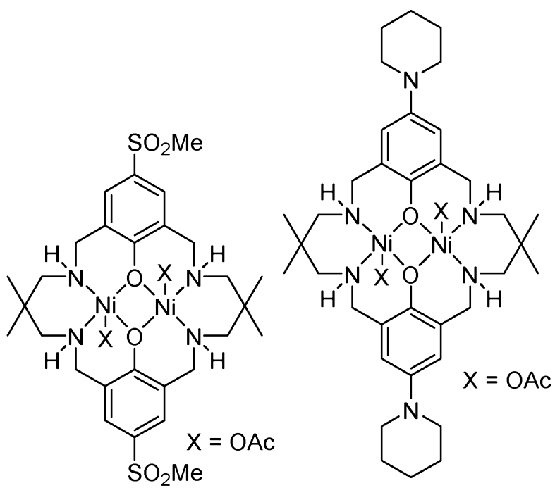
[L^7Ni_2(OAc)_2]
