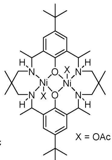
[L^4Ni_2(OAc)_2]
