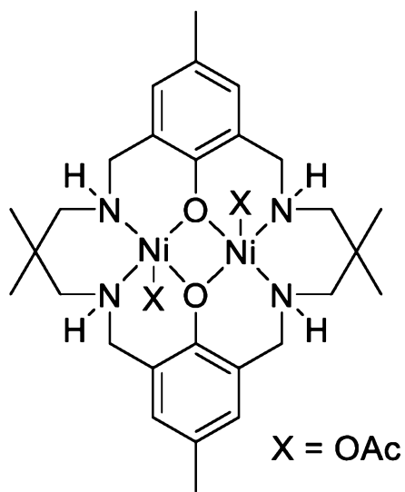
[L^2Ni_2(OAc)_2]
