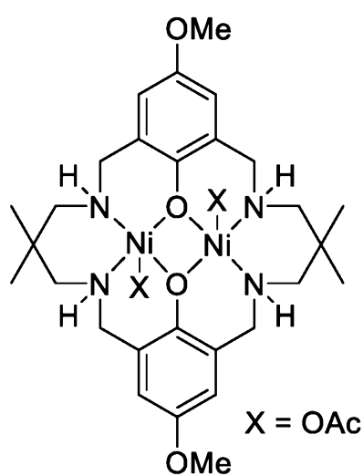
[L^3Ni_2(OAc)_2]
