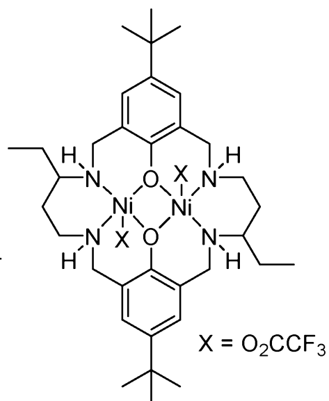
[L^{14}Ni_2(O_2CCF_3)_2]
