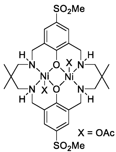
[L^7Ni_2(OAc)_2]
