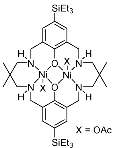
[L^5Ni_2(OAc)_2]
