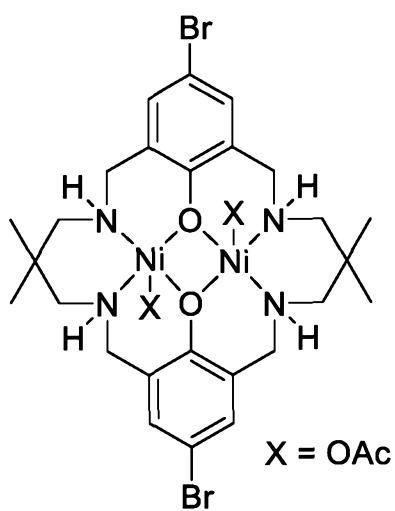
[L^6Ni_2(OAc)_2]
