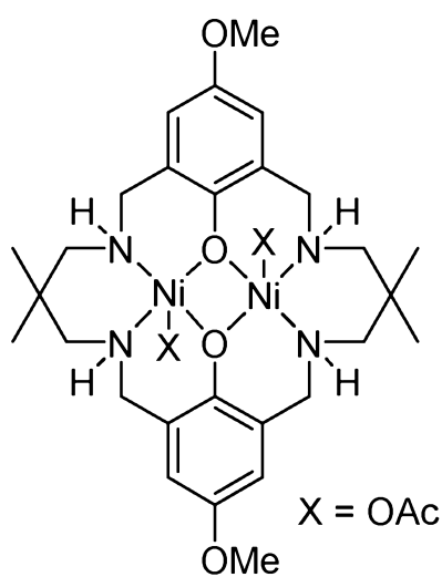
[L^3Ni_2(OAc)_2]
