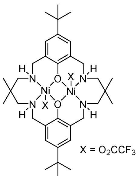
[L^1Ni_2(O_2CCF_3)_2]
