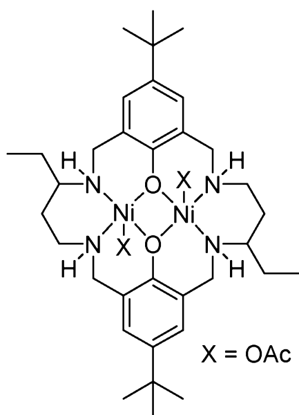
[L^{14}Ni_2(OAc)_2]
