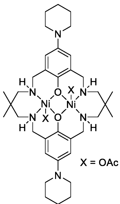
[L^8Ni_2(OAc)_2]
