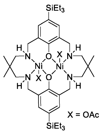
[L^5Ni_2(OAc)_2]
