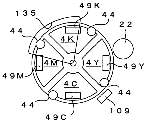
FIG. 5A : HOME POSITION
