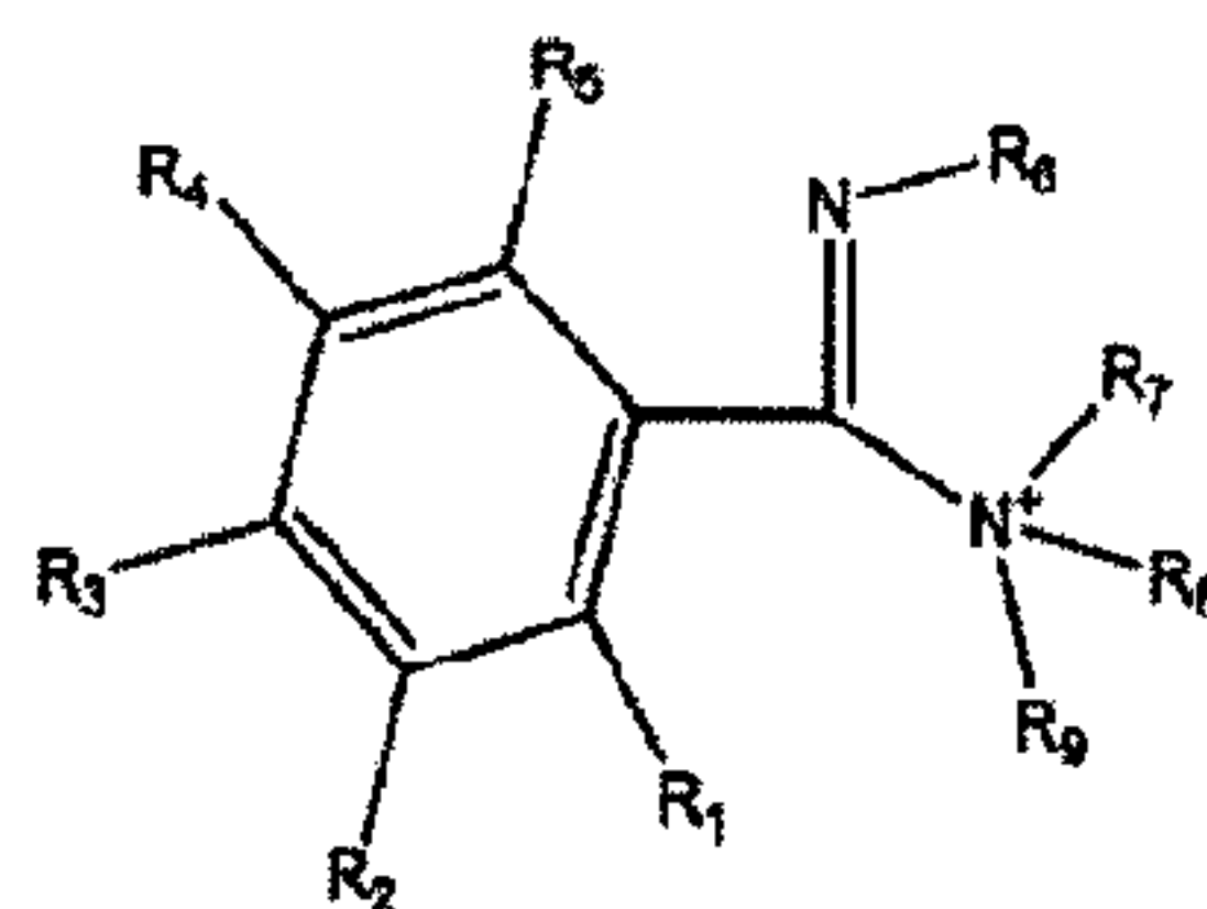
benzamidines
