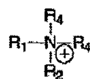
ammonium
