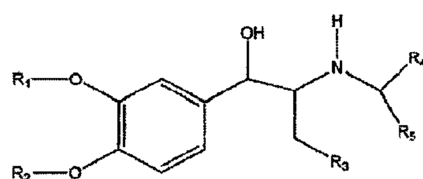
isoetarinines
