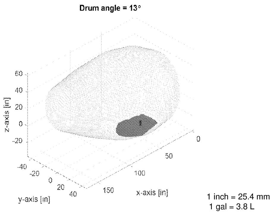
FIG. 11b
