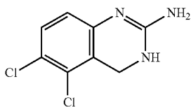
2-amino-5,6-dichloro-3,4-dihydroquinazoline
