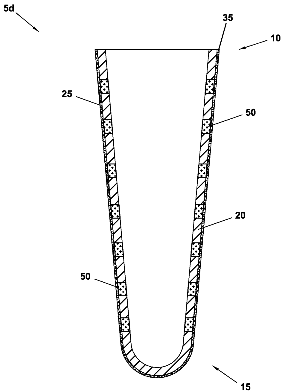
SECTION A-A
