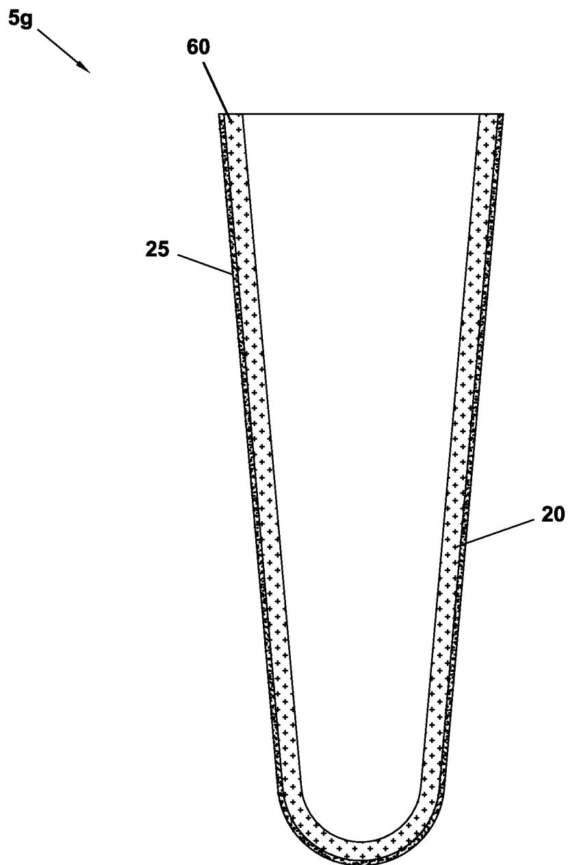
SECTION A-A
