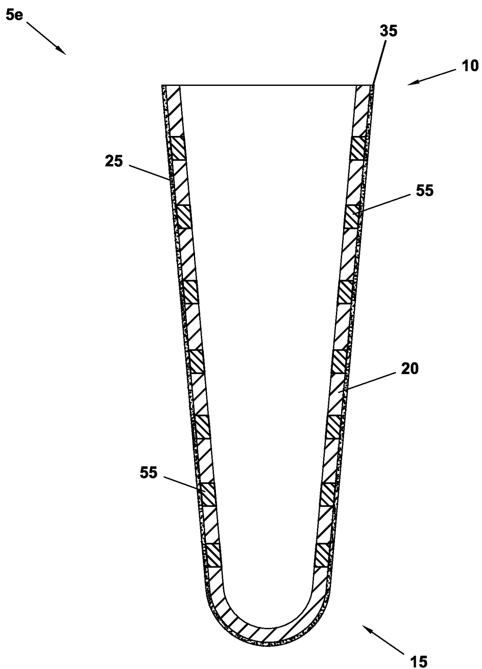
SECTION A-A
