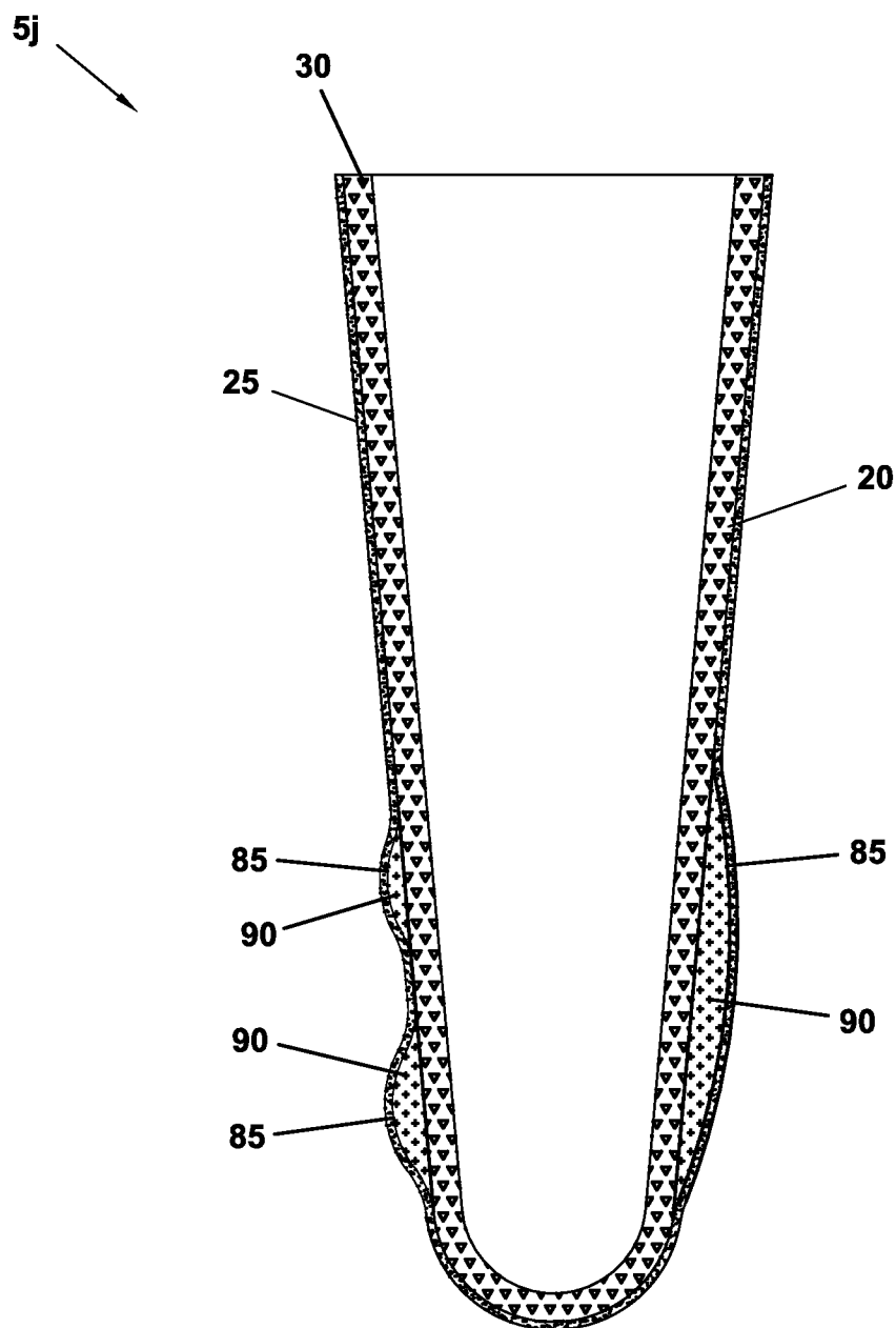
SECTION A-A
