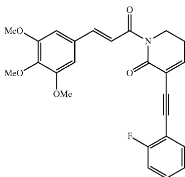
(E)-3-((2-fluorophenyl)ethynyl)-1-(3-(3,4,5-trimethoxyphenyl)prop-2-en-1-yl)-5,6-dihydropyridin-2(1H)-one
