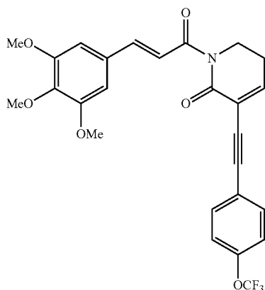
(E)-3-((4-(trifluoromethoxy)phenyl)ethynyl)-1-(3,4,5-trimethoxyphenyl)prop-2-en-1-one ridin-2(1H)-one
