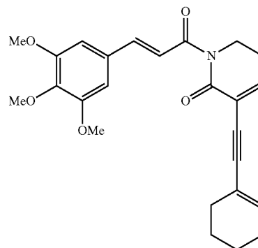
(E)-3-((cyclohexenylethynyl)-1-(3,4,5-trimethoxyphenyl)prop-2-en-1-one one
