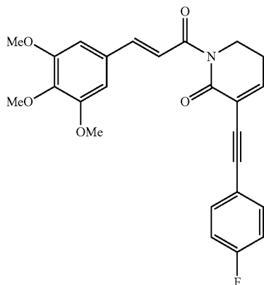
(E)-3-((4-fluorophenyl)ethynyl)-1-(3,4,5-trimethoxyphenyl)prop-2-en-1-one (1H)-one
