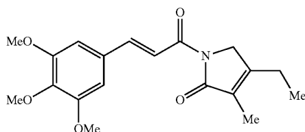
3-ethyl-4-methyl-1-[(2E)-3-(3,4,5-trimethoxyphenyl)prop-2-enoyl]-1,5-dihydro-2H-pyrrol-2-one
