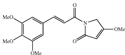
4-methoxy-1-[(2E)-3-(3,4,5-trimethoxyphenyl)prop-2-enoyl]-1,5-dihydro-2H-pyrrol-2-one
