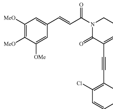
(E)-3-((2-chlorophenyl)ethynyl)-1-(3,4,5-trimethoxyphenyl)prop-2-en-1-one (1H)-one
