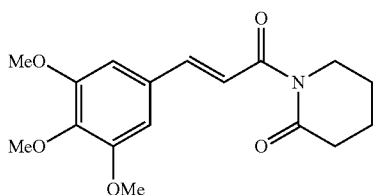
1-[(2E)-3-(3,4,5-trimethoxyphenyl)prop-2-enoyl] piperidin-2-one
