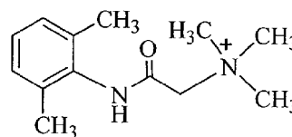
QX-222
