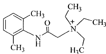
QX-314
