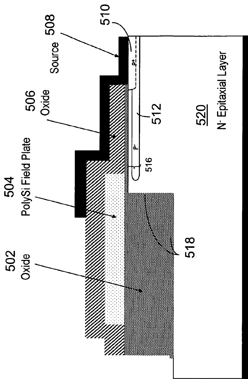
Drain FIG. 5
