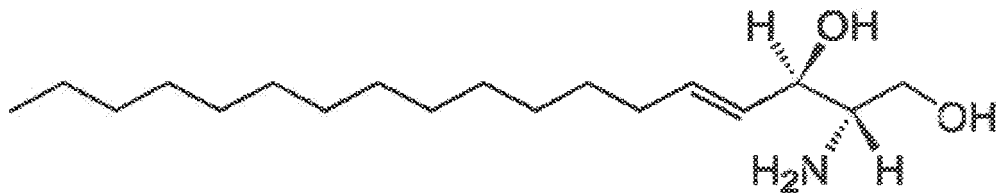
Sphingosine
