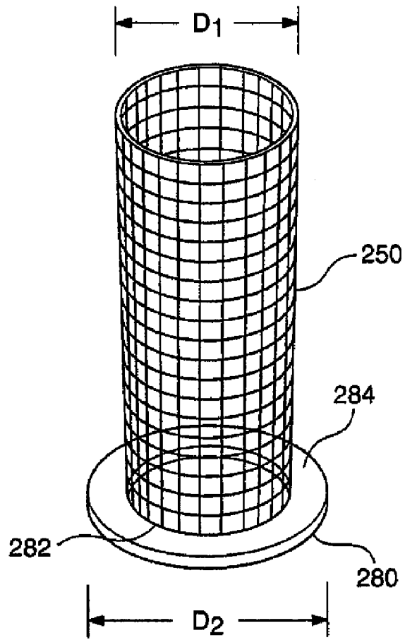
FIG. 7A
