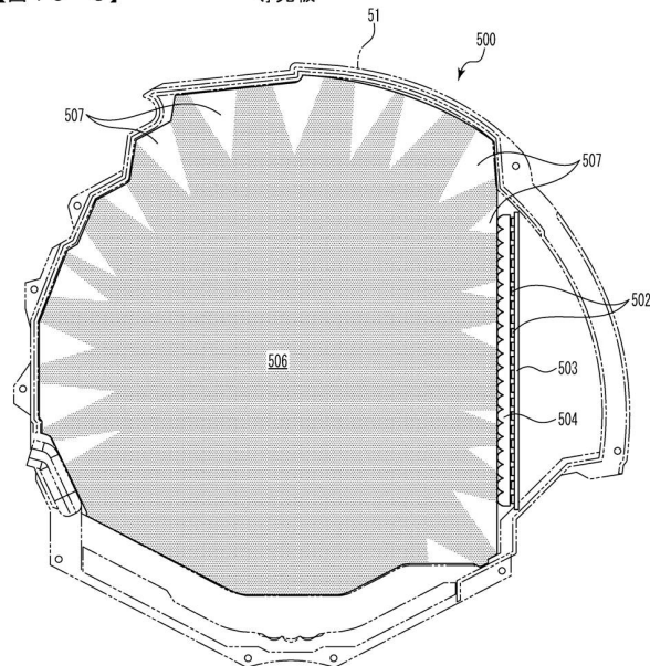
導光板
