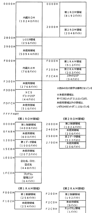
《主制御チップ全体メモリマップ》
