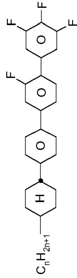
PYP-n-F
