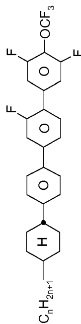
CGUQU-n-F
