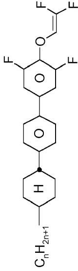
CPU-n-OXF
