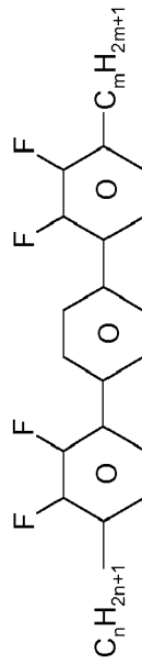
PYP-n-(O)m
