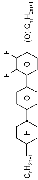
CCY-n-zOm
