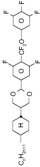
CGU-n-F
