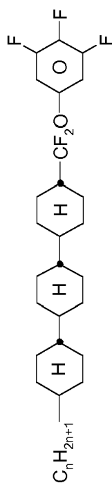
CCCQU-n-F
