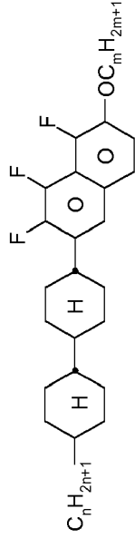
CBC-nmF
