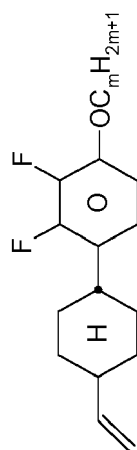
CY-V-Om
