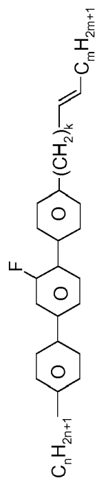
GPQU-n-F
