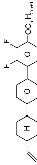
CCOC-n-m
