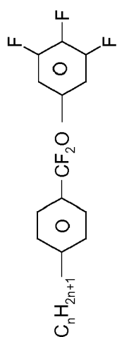
PQU-n-F
