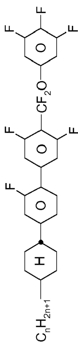
CCCQU-n-F
