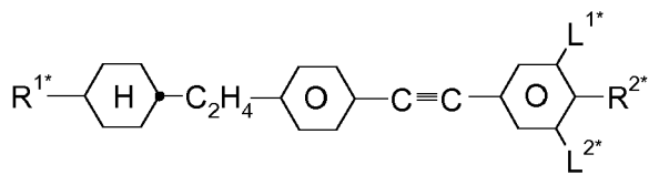
CEPTP
