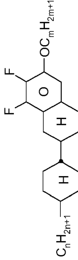
CCNap-n-Om
