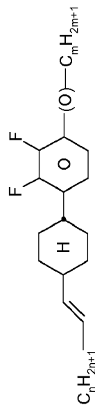
CY-nV-(O)m
