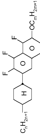
CBC-nm
