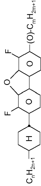
CK-n-F
