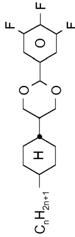
CDUQU-n-F
