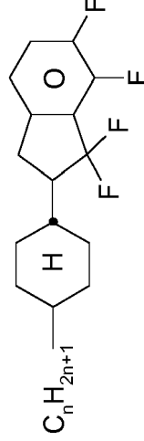
CTNap-n-Om
