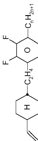
CVC-n-m
