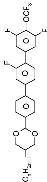
CCQG-n-F
