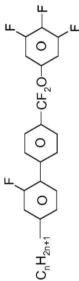
PGUQU-n-F
