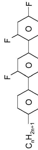
LYLI-n-m
