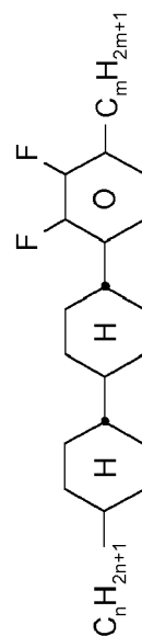
CCP-V-m
