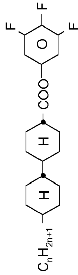
CCZU-n-F
