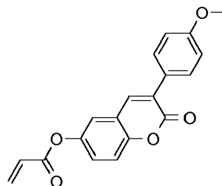
RM-15
