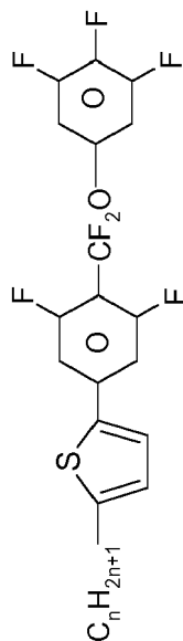
GGP-n-F
