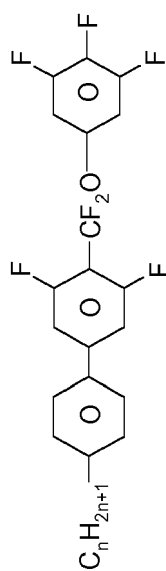
PUQU-n-F
