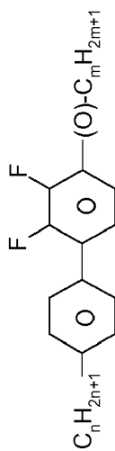
CVY-V-m
