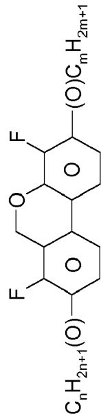
CETNap-n-Om
