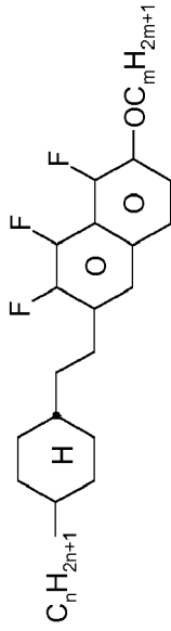
Cnap-n-Om
