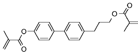
RM-6
