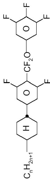
CUQU-n-F
