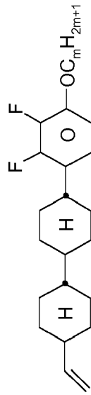
CCY-V-m
