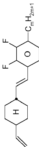
CY-nV-(O)m
