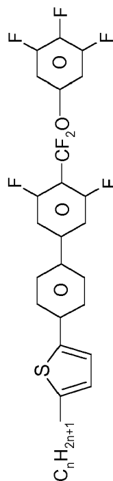
SPUQU-n-F
