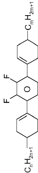
CLY-n-(O)m
