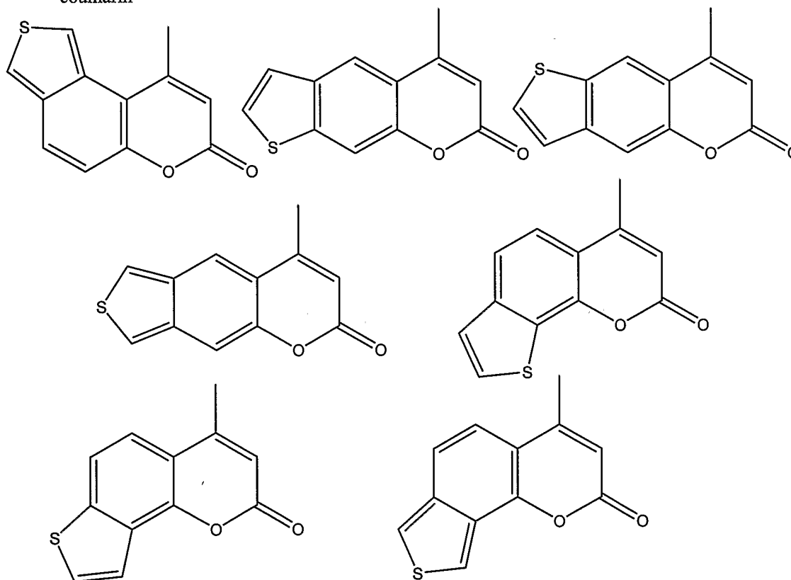
coumarin
