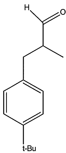
lilial
