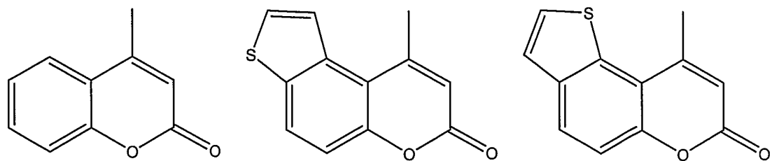
coumarin
