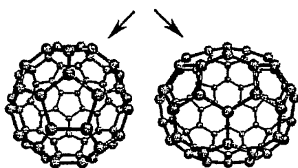
C 60 (I h )
