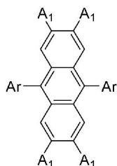
化学式 4
