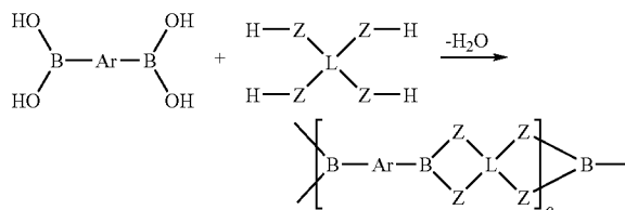
Scheme 1a
