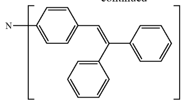
Dotand D1
