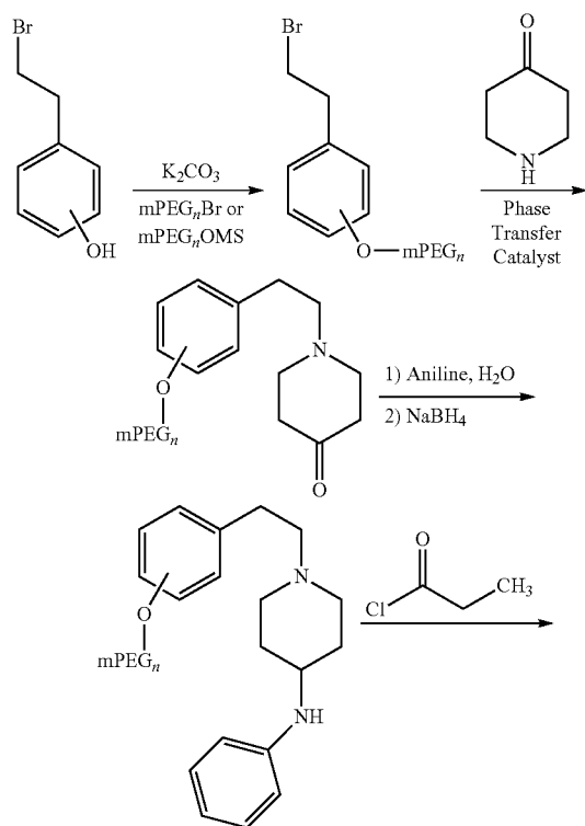
Scheme 11-A
