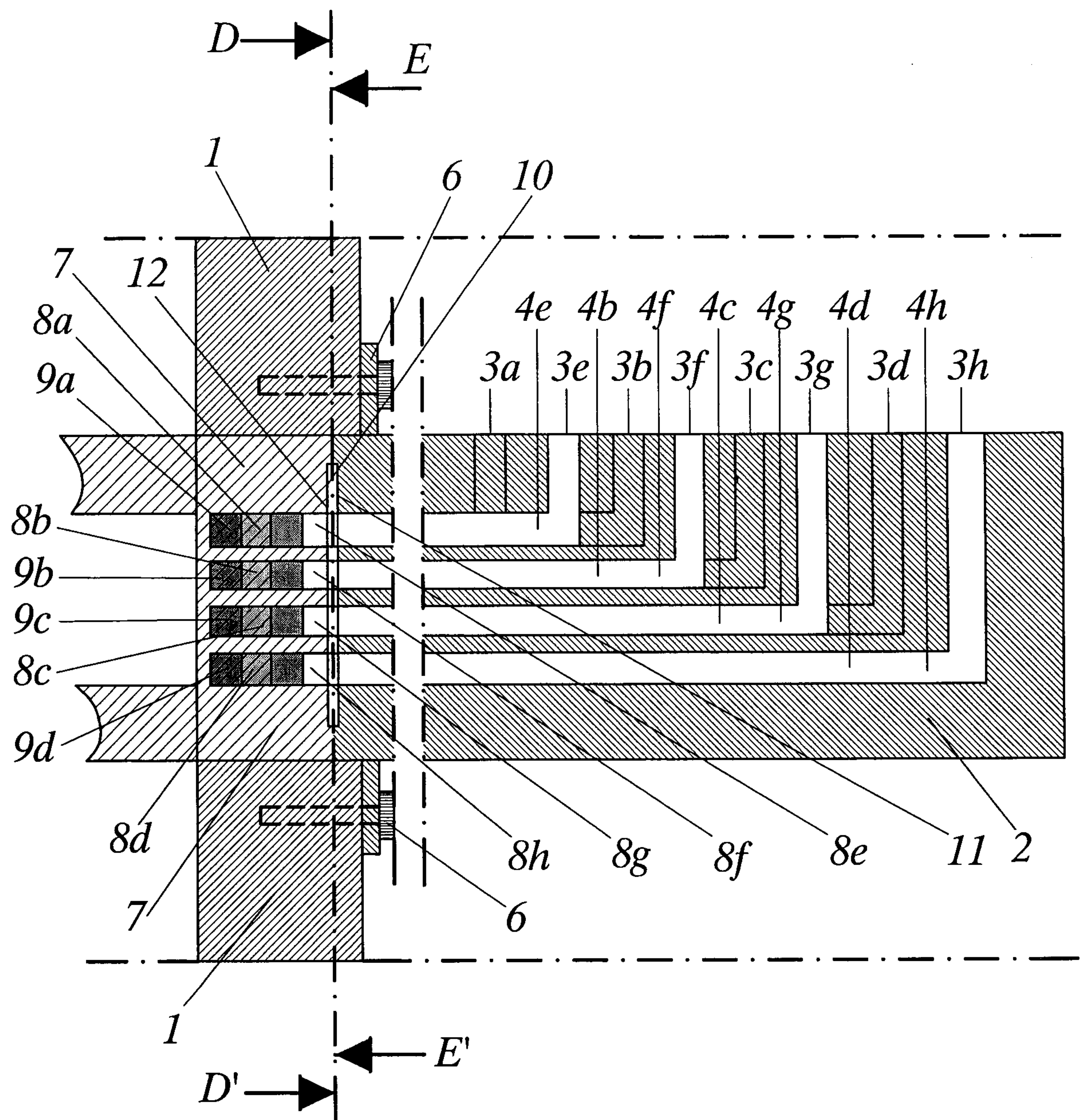
FIG. 3 (B-B')
