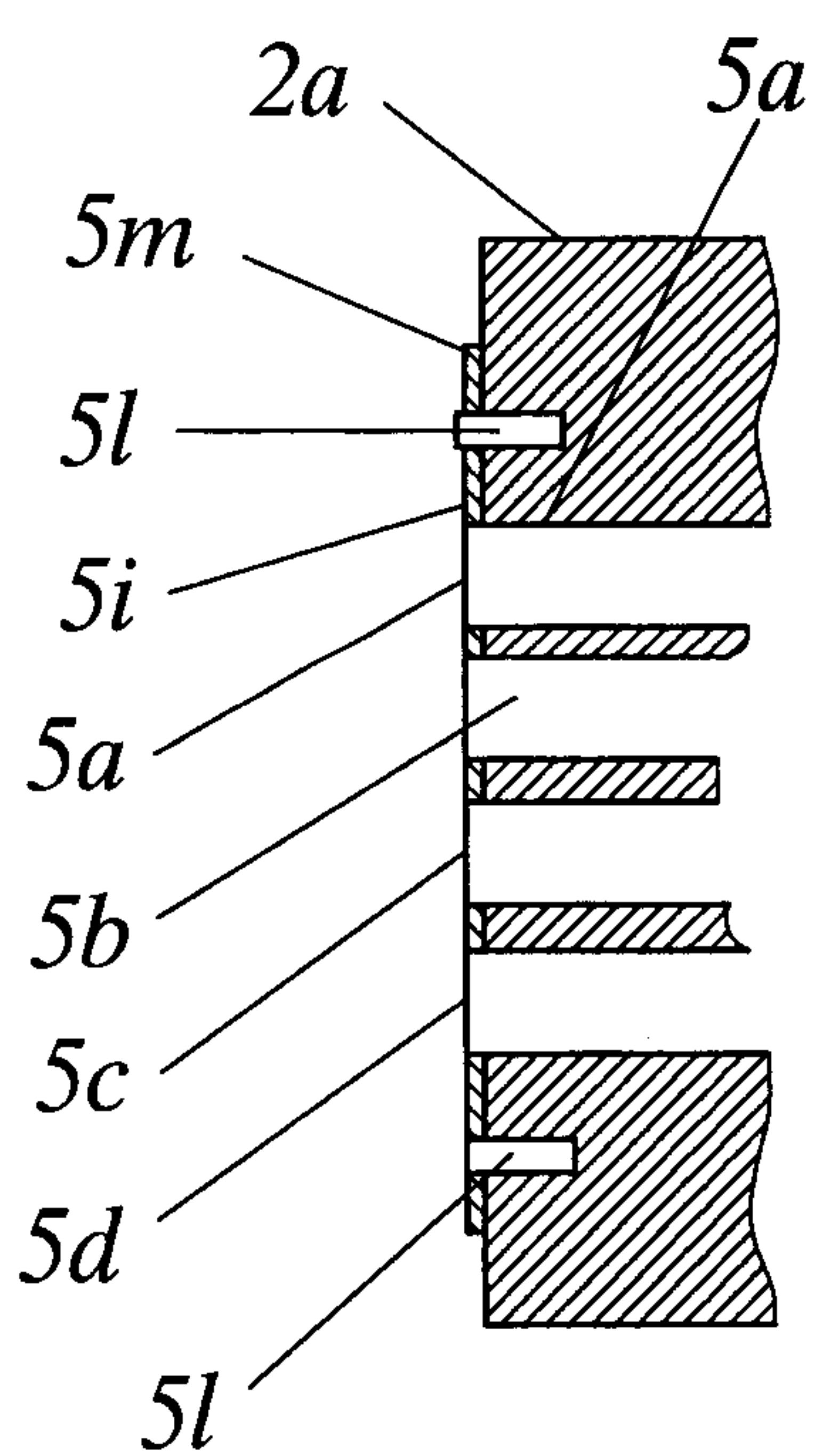
FIG. 15 (H-H)
