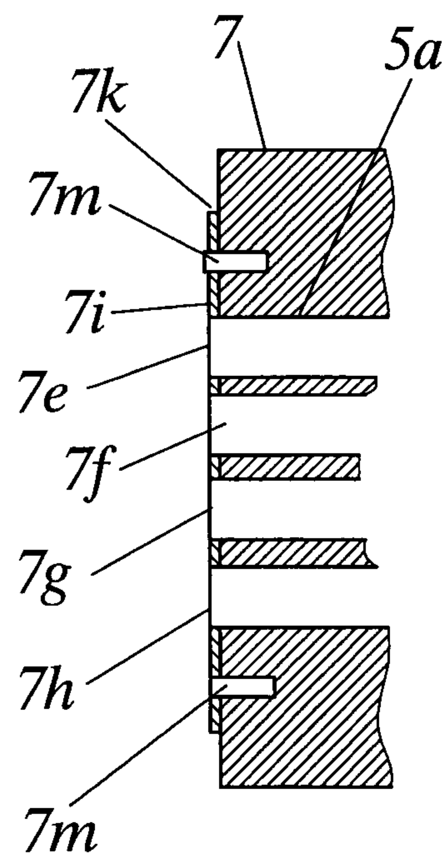
FIG. 12 (G-G')
