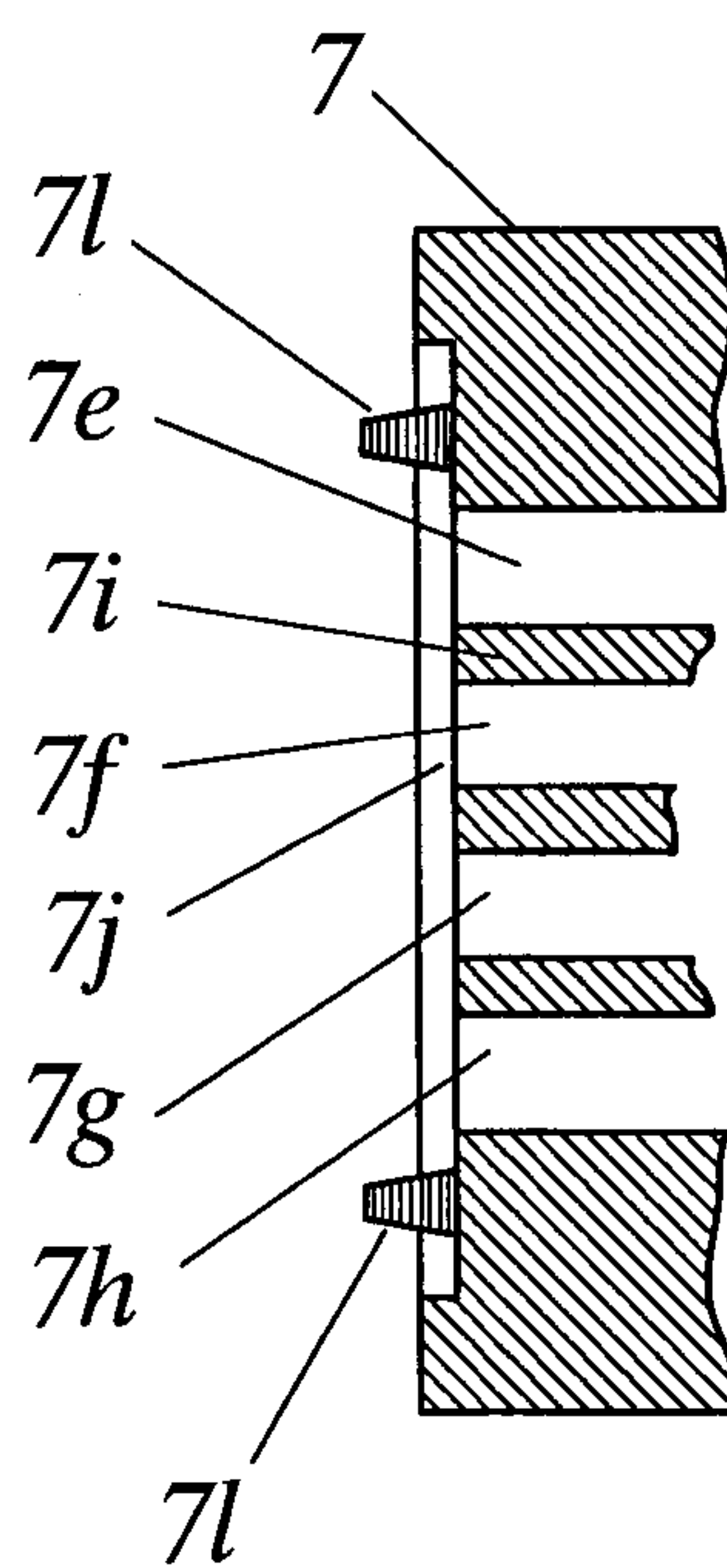
FIG. 16 (I-I)
