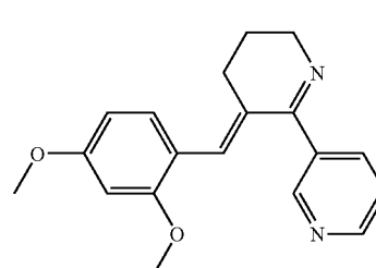
3-(2,4-dimethoxybenzylidene) anabaseine
