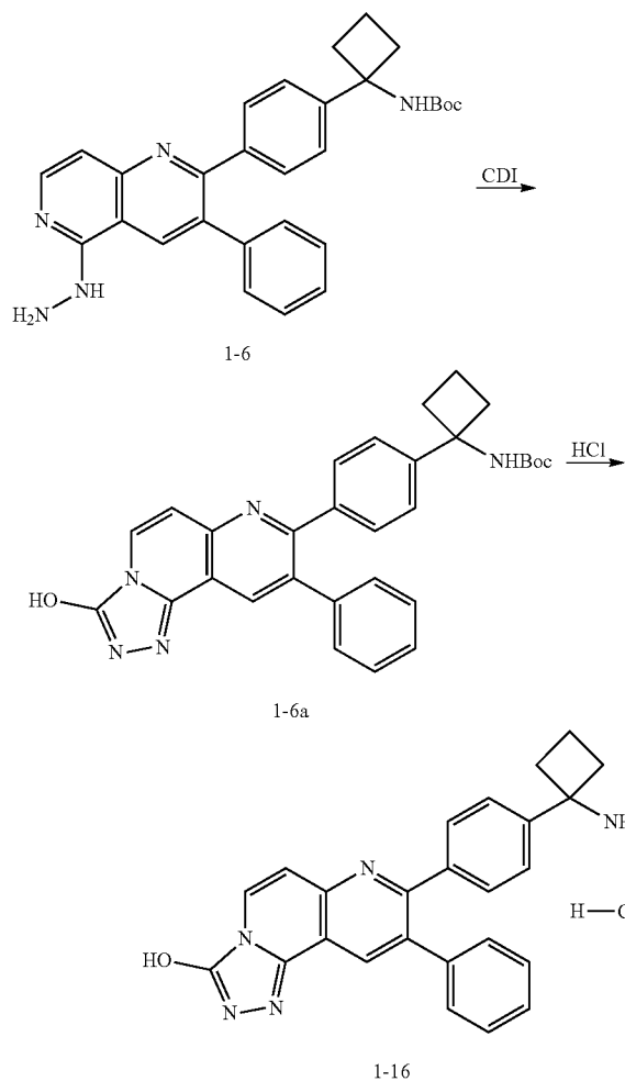
SCHEME 1A
