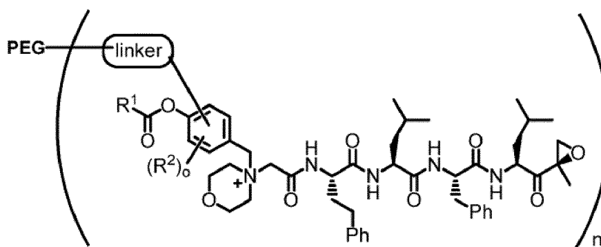
Formule I
