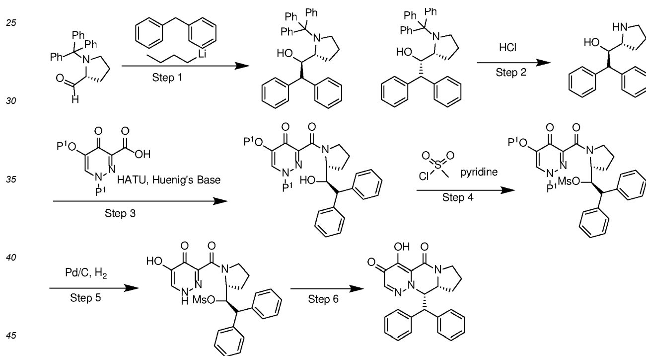
Scheme B.
