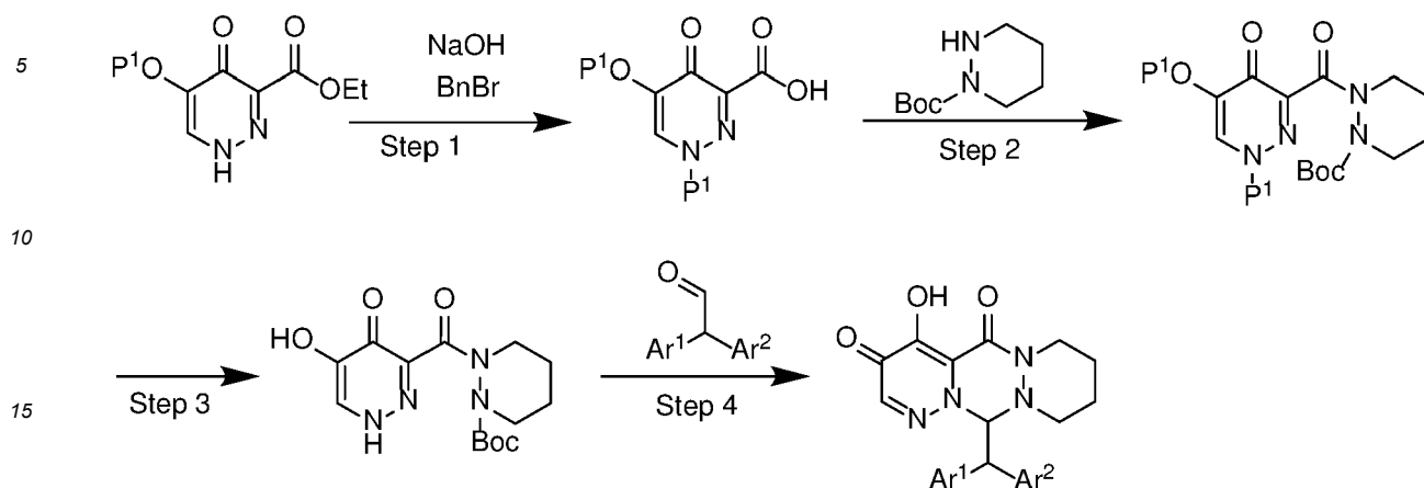
Scheme A.
