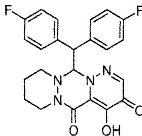
1a 12-(bis(4-fluorophényl)méthyl)-4-hydroxy-7,8,9,10-tétrahydro-12H-dipyridazino[1,2-a:1',6'-d][1,2,4]triazine-3,5-dione ;
