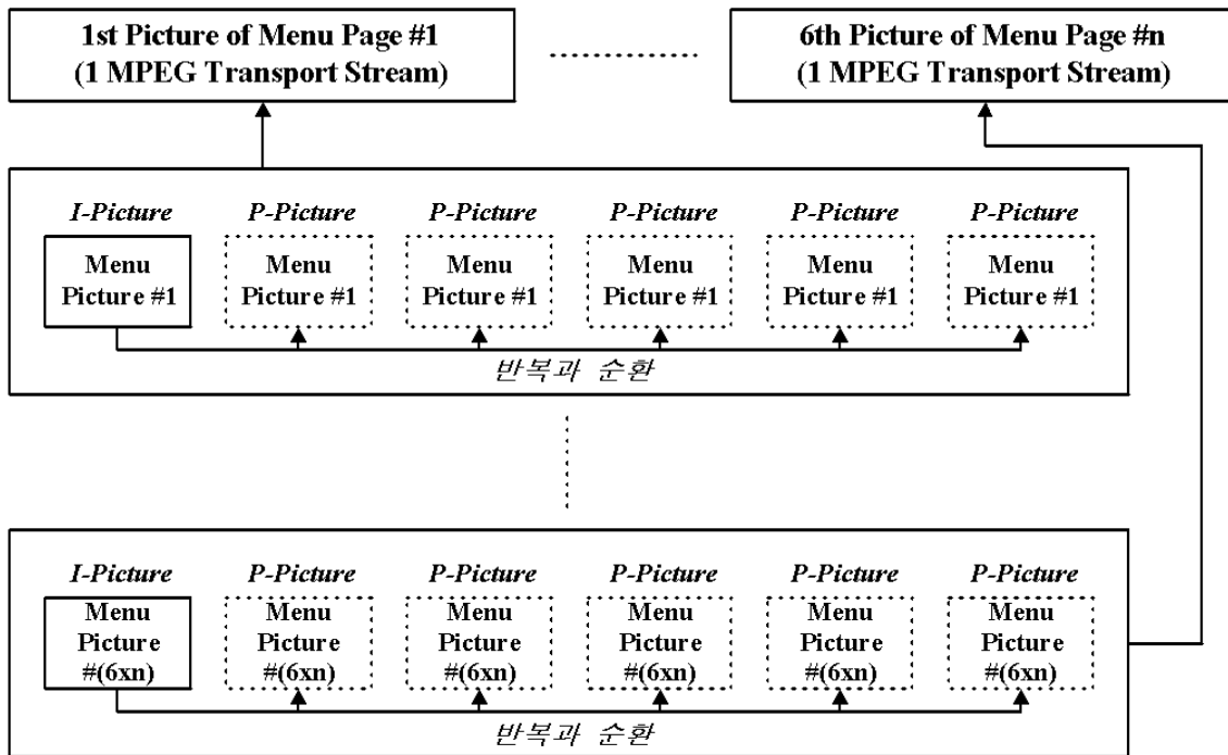
VSB 변조를 통한 메뉴데이터 전송방법
