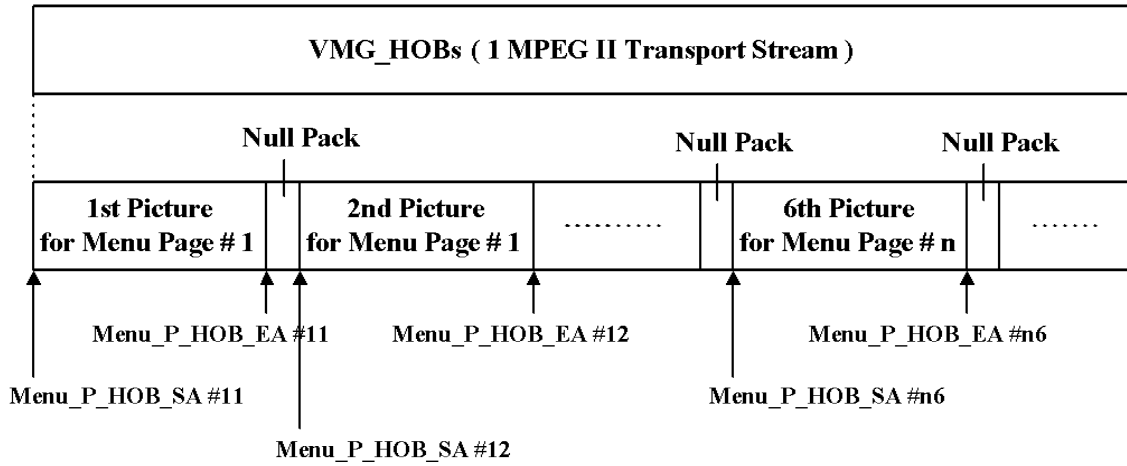
VSB 변조 전송방식에 대한 메뉴데이터 스트림의 구조
