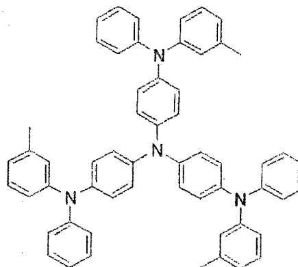
m-MTDATA : E_a=1.9 , I_p=5.1
