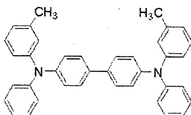
TPD : E_a=2.3 , I_p=5.5
