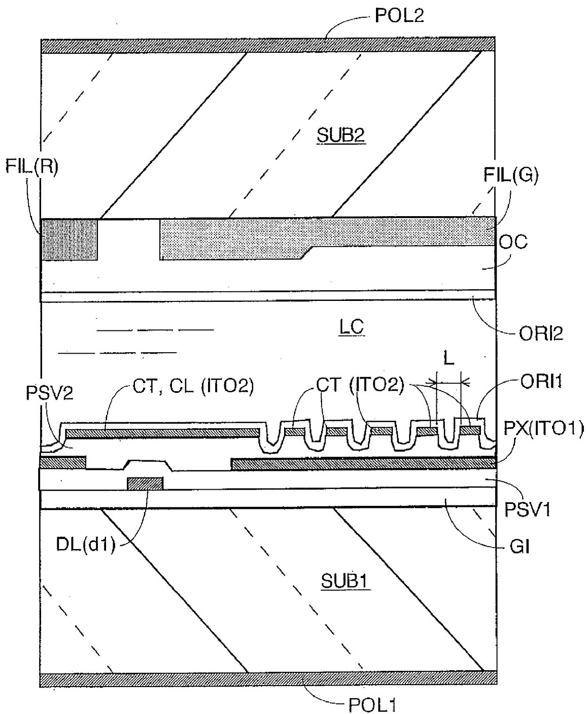
FIG. 43
