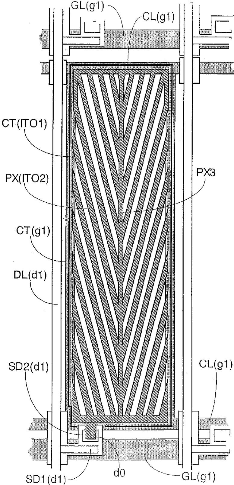
FIG. 48
