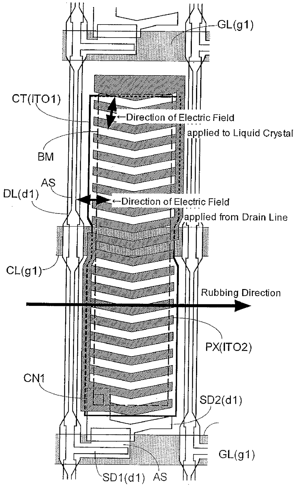
FIG. 50
