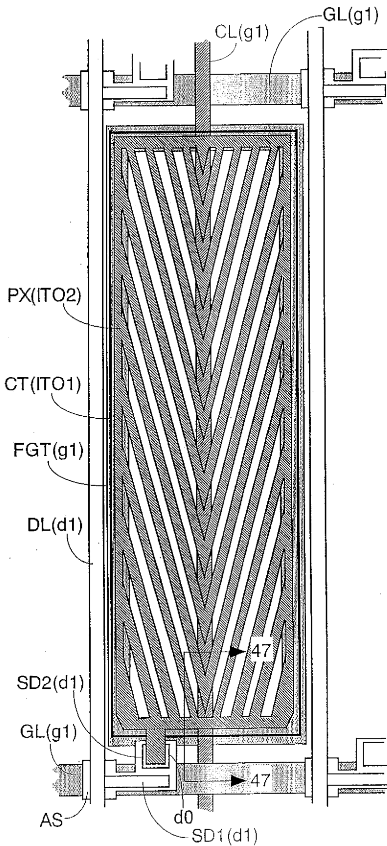
FIG. 46
