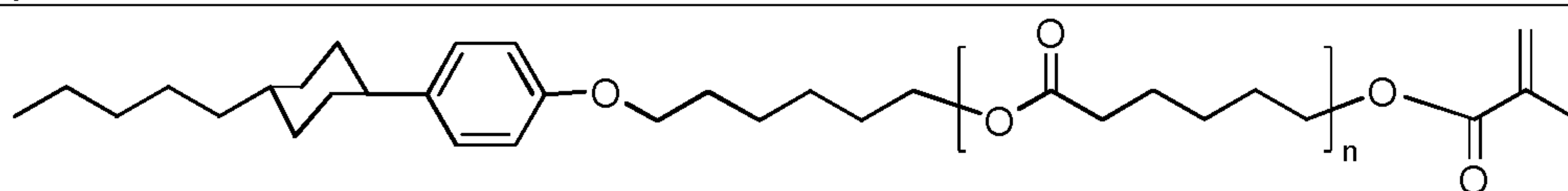
1-(6-(6-(6-(6-(6-(6-(4-(4-(trans-4-pentylcyclohexyl)phenoxy)carbonyl)phenoxy)hexyloxy)-6-oxohexyloxy)-6-oxohexyloxy)-6-oxohexyloxy)-6-oxohexyloxy)-6-oxohexyloxy)-2-methylprop-2-en-1-one
