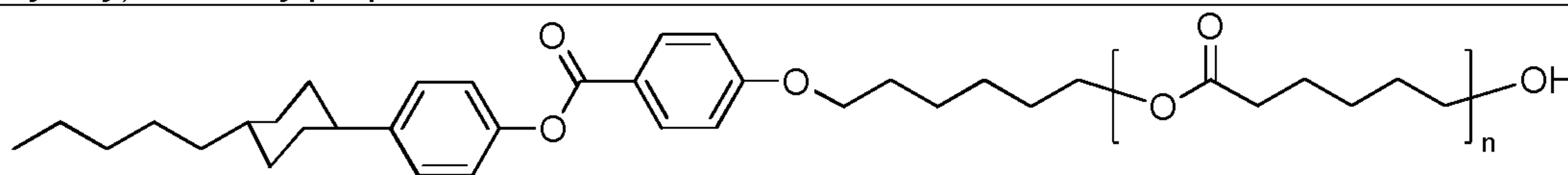
1-(6-(6-(6-(6-(4-(4-(trans-4-pentylcyclohexyl)phenoxy)hexyloxy)-6-oxohexyloxy)-6-oxohexyloxy)-6-oxohexyloxy)-2-methylprop-2-en-1-one
