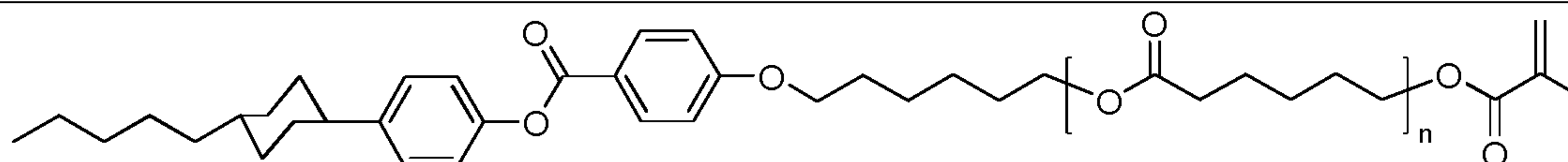
1-(6-(6-(6-(6-(4-(4-(trans-4-pentylcyclohexyl)phenoxy)carbonyl)phenoxy)hexyloxy)-6-oxohexyloxy)-6-oxohexyloxy)-2-methylprop-2-en-1-one
