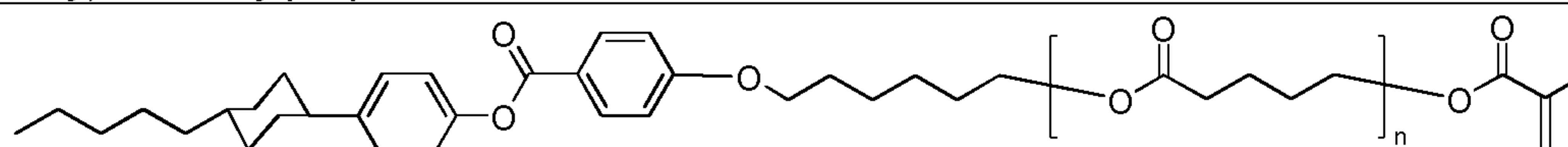
1-(6-(6-(6-(6-(6-(6-(6-(4-(4-(trans-4-pentylcyclohexyl)phenoxy)carbonyl)phenoxy)hexyloxy)-6-oxohexyloxy)-6-oxohexyloxy)-6-oxohexyloxy)-6-oxohexyloxy)-6-oxohexyloxy)-2-methylprop-2-en-1-one
