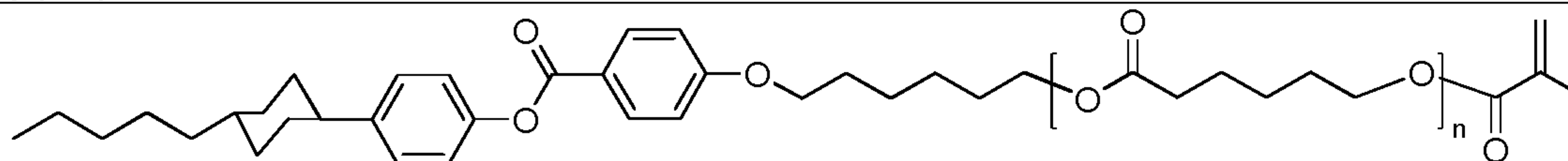
1-(6-(6-(6-(6-(6-(6-(6-(6-(6-(6-(4-(4-(trans-4-pentylcyclohexyl)phenoxy)carbonyl)phenoxy)hexyloxy)-6-oxohexyloxy)-6-oxohexyloxy)-6-oxohexyloxy)-6-oxohexyloxy)-6-oxohexyloxy)-6-oxohexyloxy)-2-methylprop-2-en-1-one
