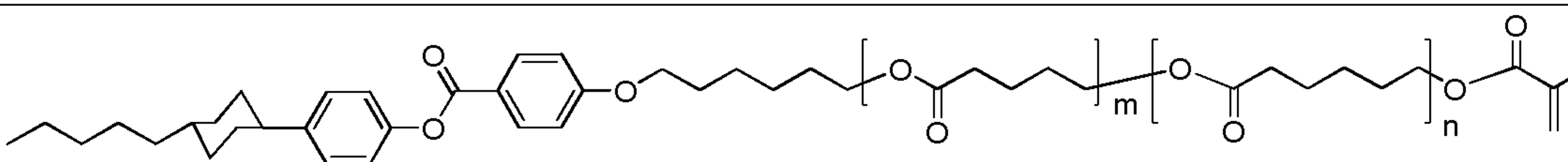
1-(6-(6-(6-(6-(6-(6-(6-(6-(6-(6-(6-(6-(6-(6-(6-(6-(4-(4-(trans-4-pentylcyclohexyl)phenoxy)carbonyl)phenoxy)hexyloxy)-6-oxohexyloxy)-6-oxohexyloxy)-6-oxohexyloxy)-6-oxohexyloxy)-6-oxohexyloxy)-6-oxohexyloxy)-6-oxohexyloxy)-6-oxohexyloxy)-6-oxohexyloxy)-2-methylprop-2-en-1-one
