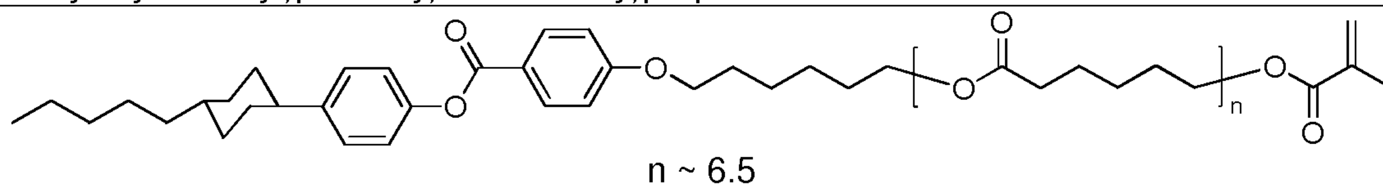
1-(6-(6-(6-(6-(6-(6-(4-(4-(trans-4-pentylcyclohexyl)phenoxy)carbonyl)phenoxy)hexyloxy)-6-oxohexyloxy)-6-oxohexyloxy)-6-oxohexyloxy)-6-oxohexyloxy)-6-oxohexyloxy)-2-methylprop-2-en-1-one
