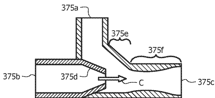
375 FIG. 5A
