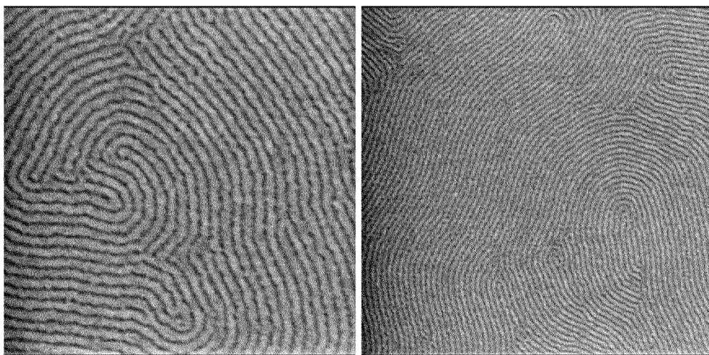
Random copolymer:
