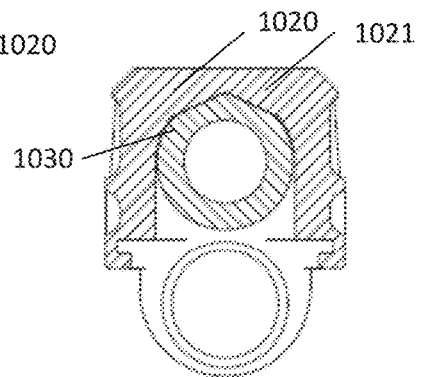
SECTION AU-AU
