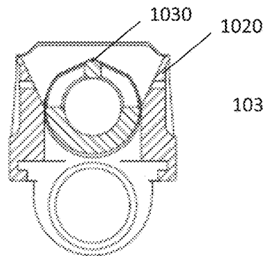
SECTION AV-AV
