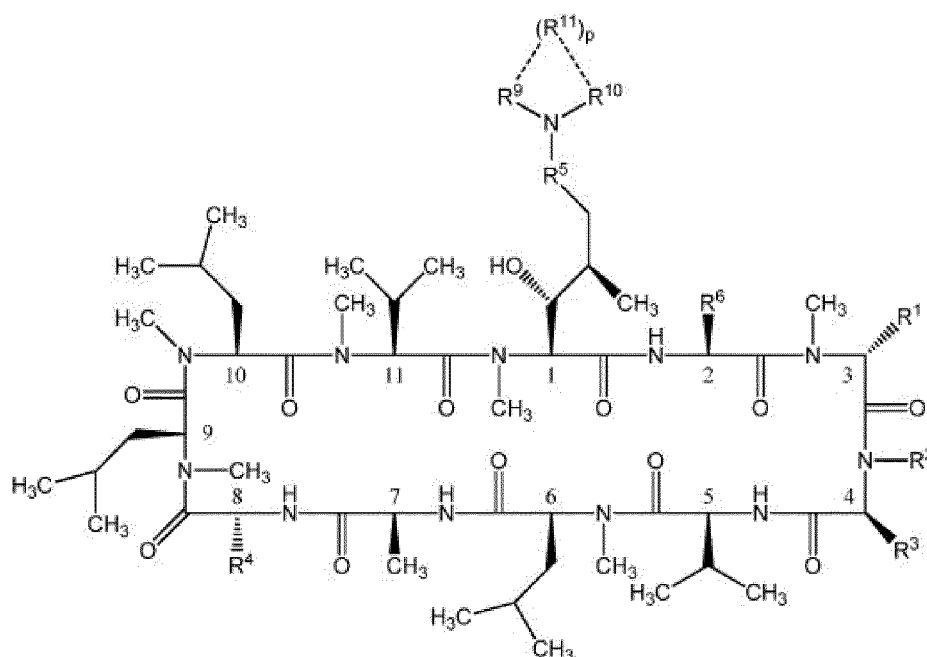
Formule I
