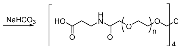
4-arm-PEG20k-CM-beta-alanine
