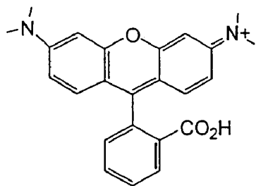
Rhodamine
