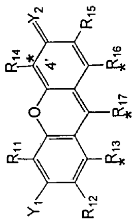
XANTHENE
