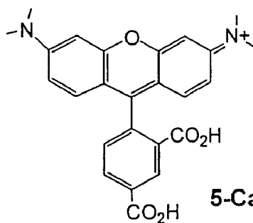
Rhodamine
