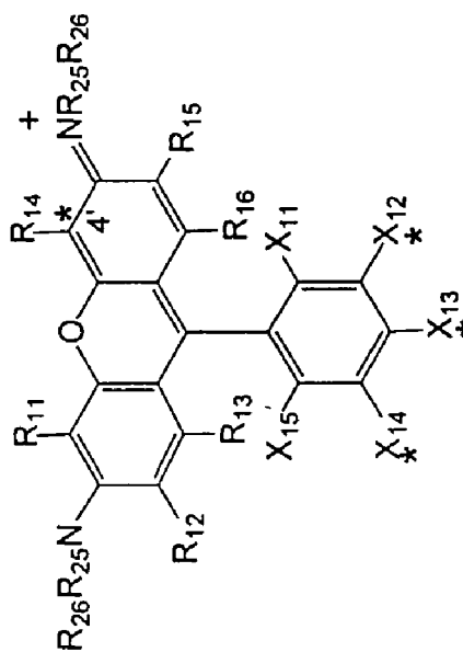
RHODAMINE
